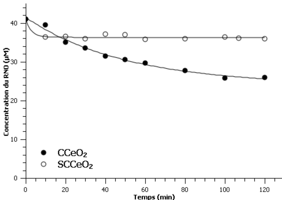
Figure 19. Blanchissement du RNO en présence de la cérine calcinée ( CCeO_2 ) et sulfatée ( SCCeO_2 ). Conditions : 1,5 g/L du catalyseur, 0,6 M d' H_2O_2 , à l'obscurité, pH = 4 et à T = 22\text{ }^\circ\text{C} .
