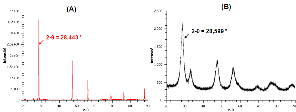
Figure 2. Diffractogrammes (A) d'une plaque de silicium et (B) de l'oxyde de cérium pur.
