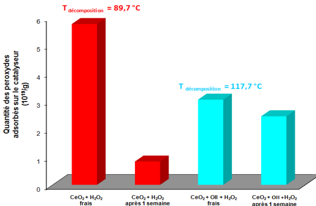
Figure 32. Stabilité des espèces peroxydes en fonction du temps en absence/présence du colorant à la surface du CeO 2 .
