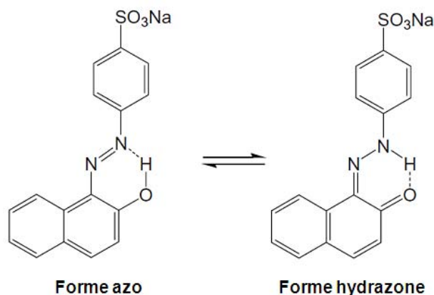
Figure 28. Les deux formes tautomères de l'Orange II.
