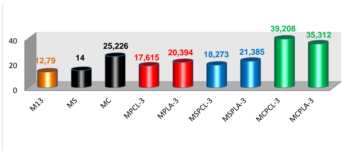
Figure III.69. Pourcentage de la perte de masse des nanocomposites-3 à base de bentonite (par polymérisation in situ)
