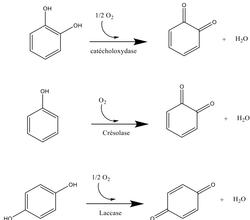
Figure 1 : Schéma des réactions catalysées par les polyphénol-oxydases (PPO) (modifié de Maghsoudi et al., 2013)
