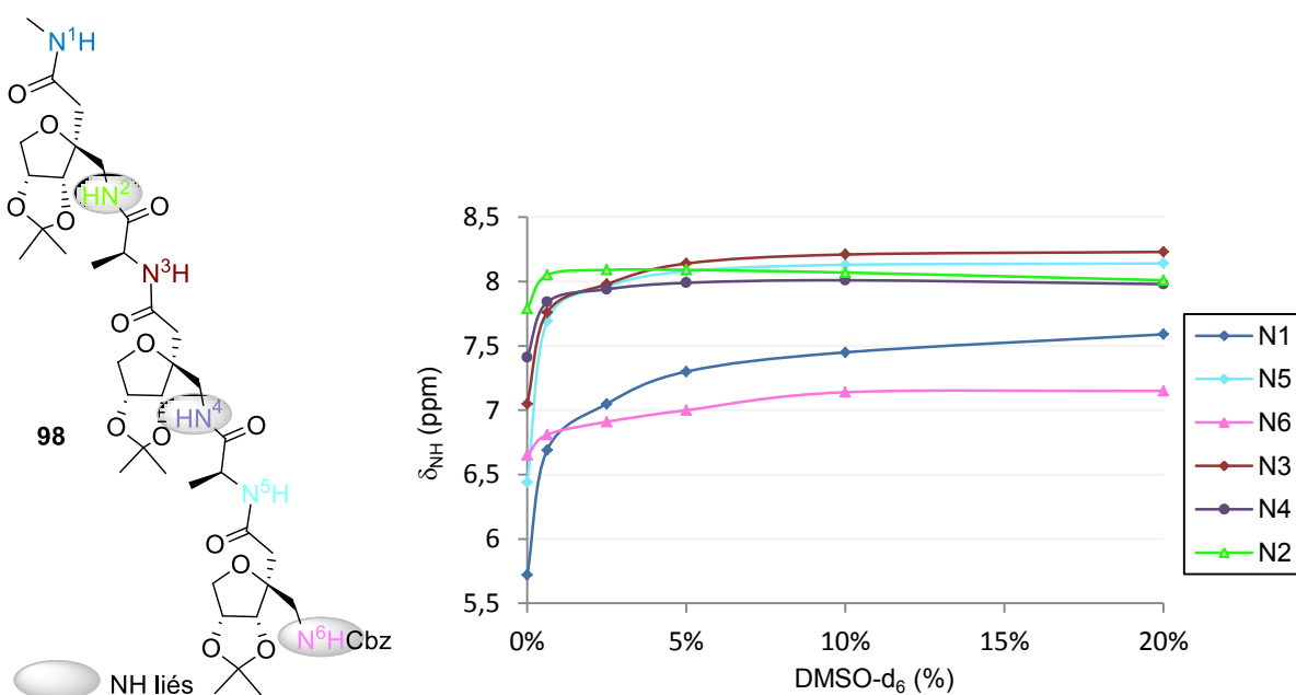
Figure 30. Courbes de titration du pentapeptide 98 entre 0 et 20% de DMSO-d 6
