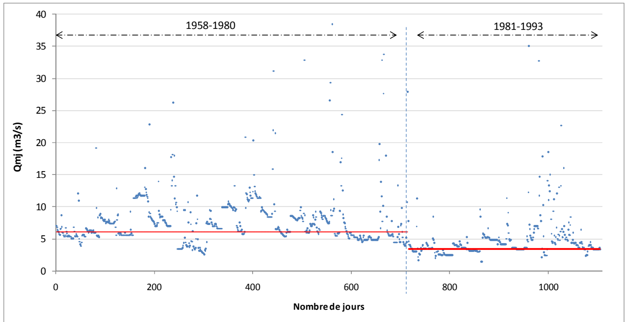
Annexe 5.6 : Hydrogramme composé des mois de septembre à la station d'Azzaba et d'El Mers et débit modal selon Fréchet (pour la station d'El Mers les valeurs supérieures à 3 ne sont pas représentées)
