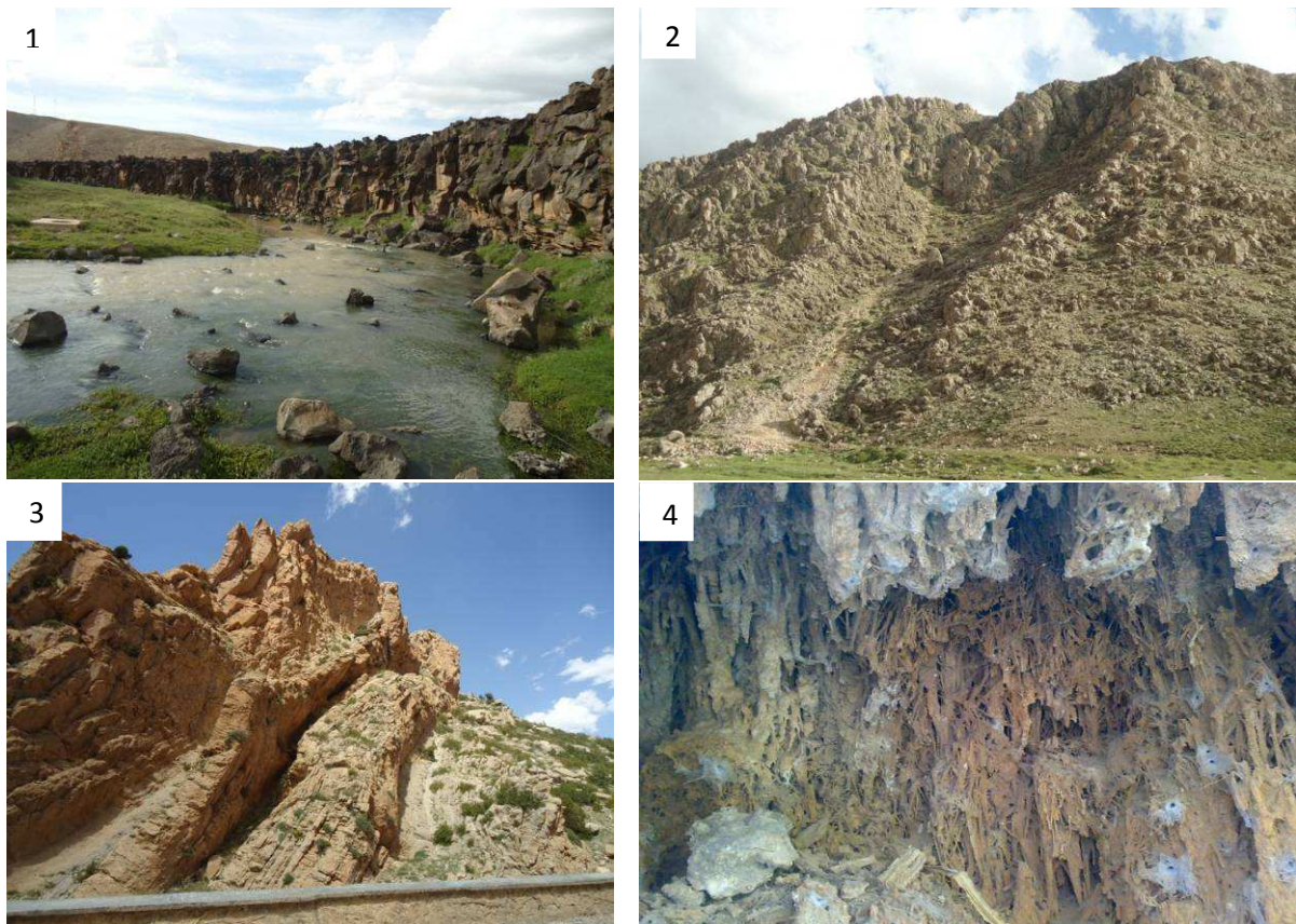
1: Basalte de Bou Anger Skoura
