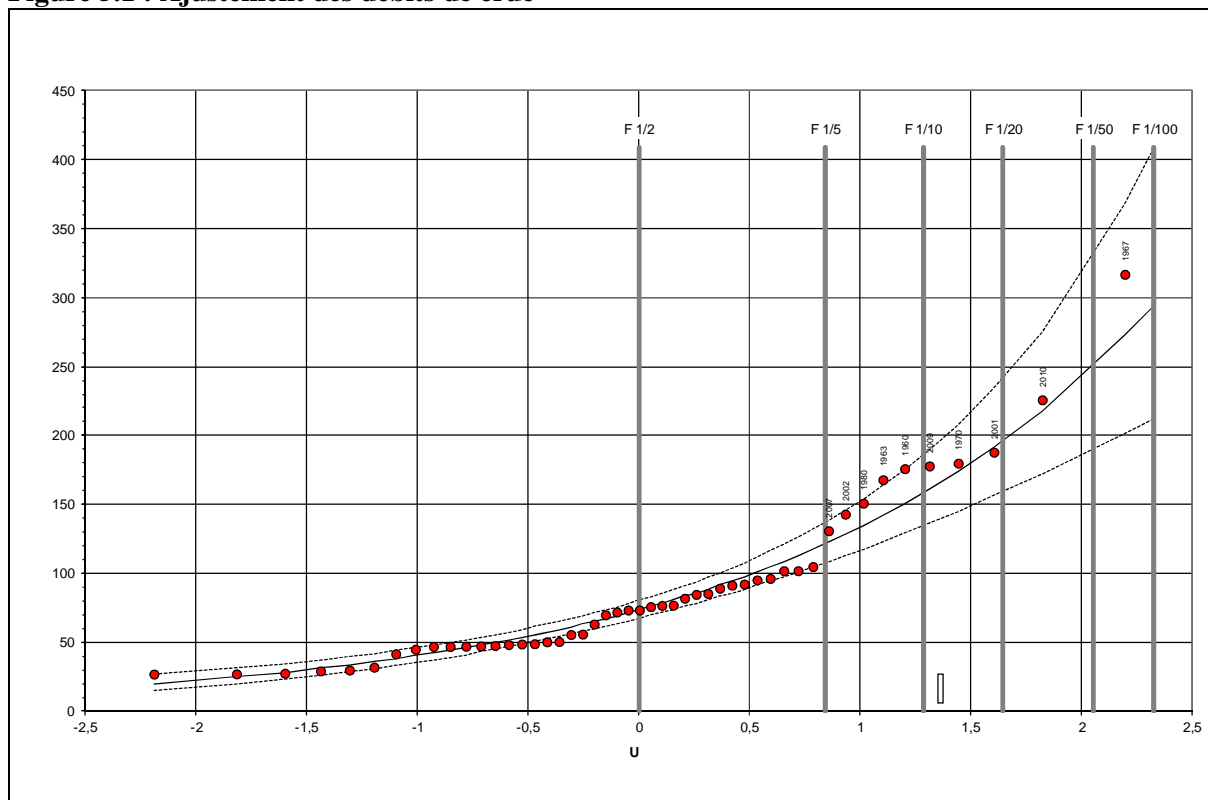
Figure 5.1 : Ajustement des débits de crue
