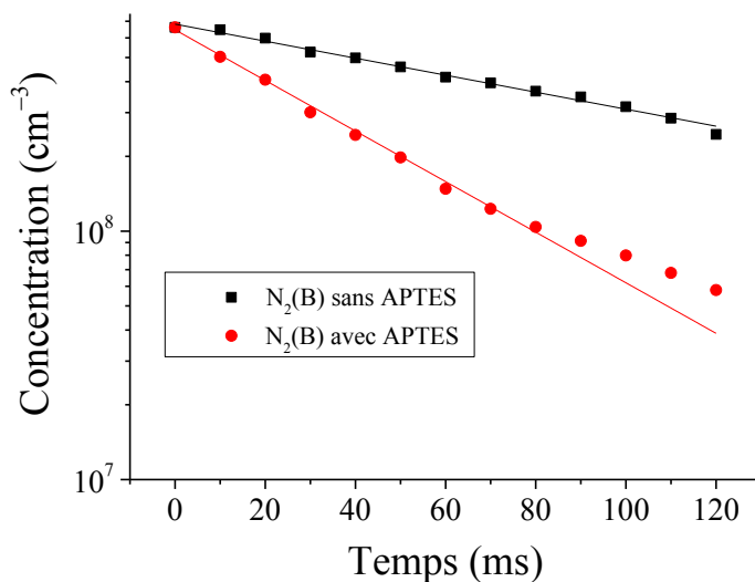
Figure 44: Evolution temporelle des concentrations de N 2 (B, v'=11) avec et sans APTES (P = 20 mbar, P w = 100 W, débit Ar = 1050 Nccm, débit N 2 = 100 Nccm, débit APTES = 0,13 Nccm).
