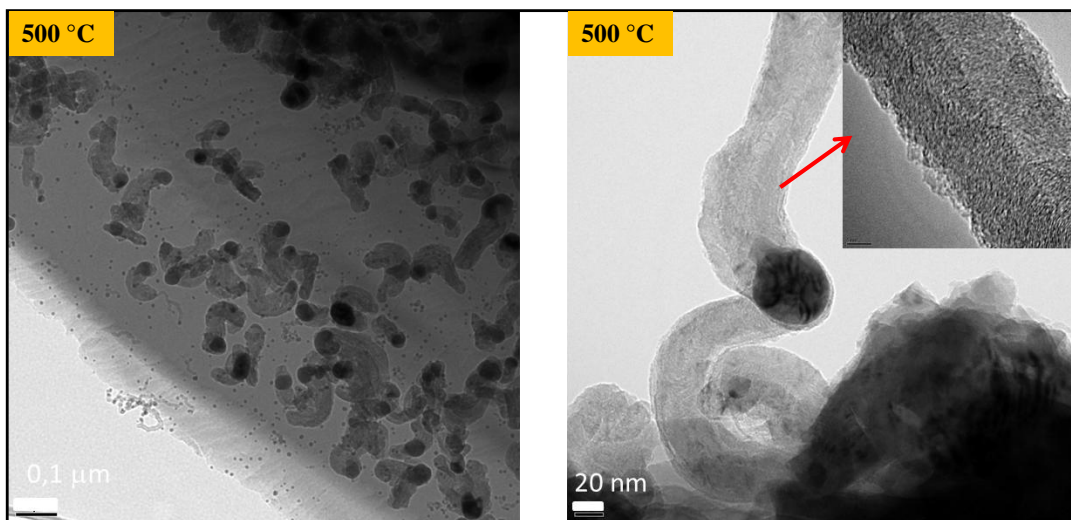
Figure 47: Images MET de l'échantillon synthétisé à 500°C sur des catalyseurs réalisés par CVD
