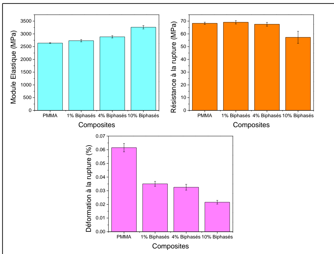
Figure 90: Comparaison des propriétés mécaniques du PMMA et du PMMA renforcé par 1, 4 et 10% de charges biphasés
