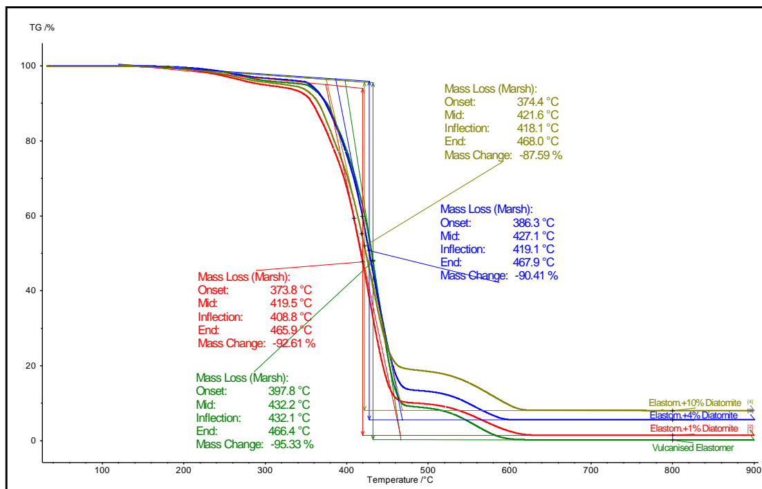
Figure 93: Degradation thermique du SBR et du SBR chargé par des diatomées
