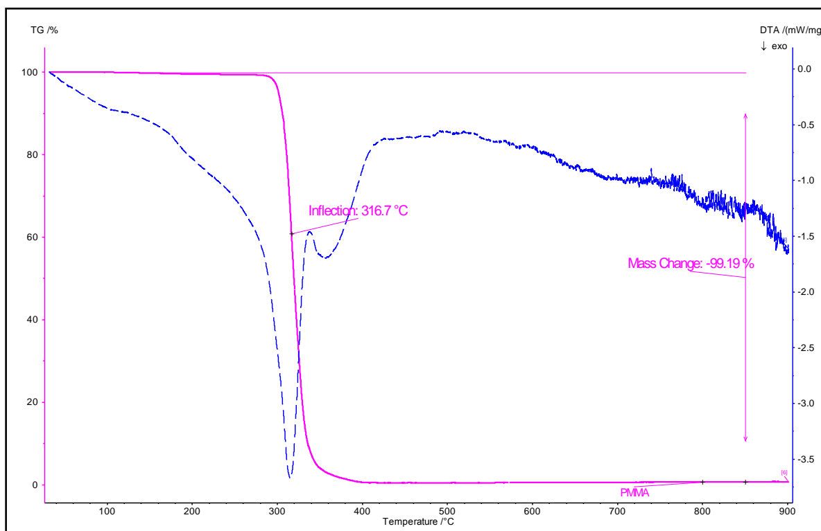
Figure 84: Dégradation thermique du PMMA
