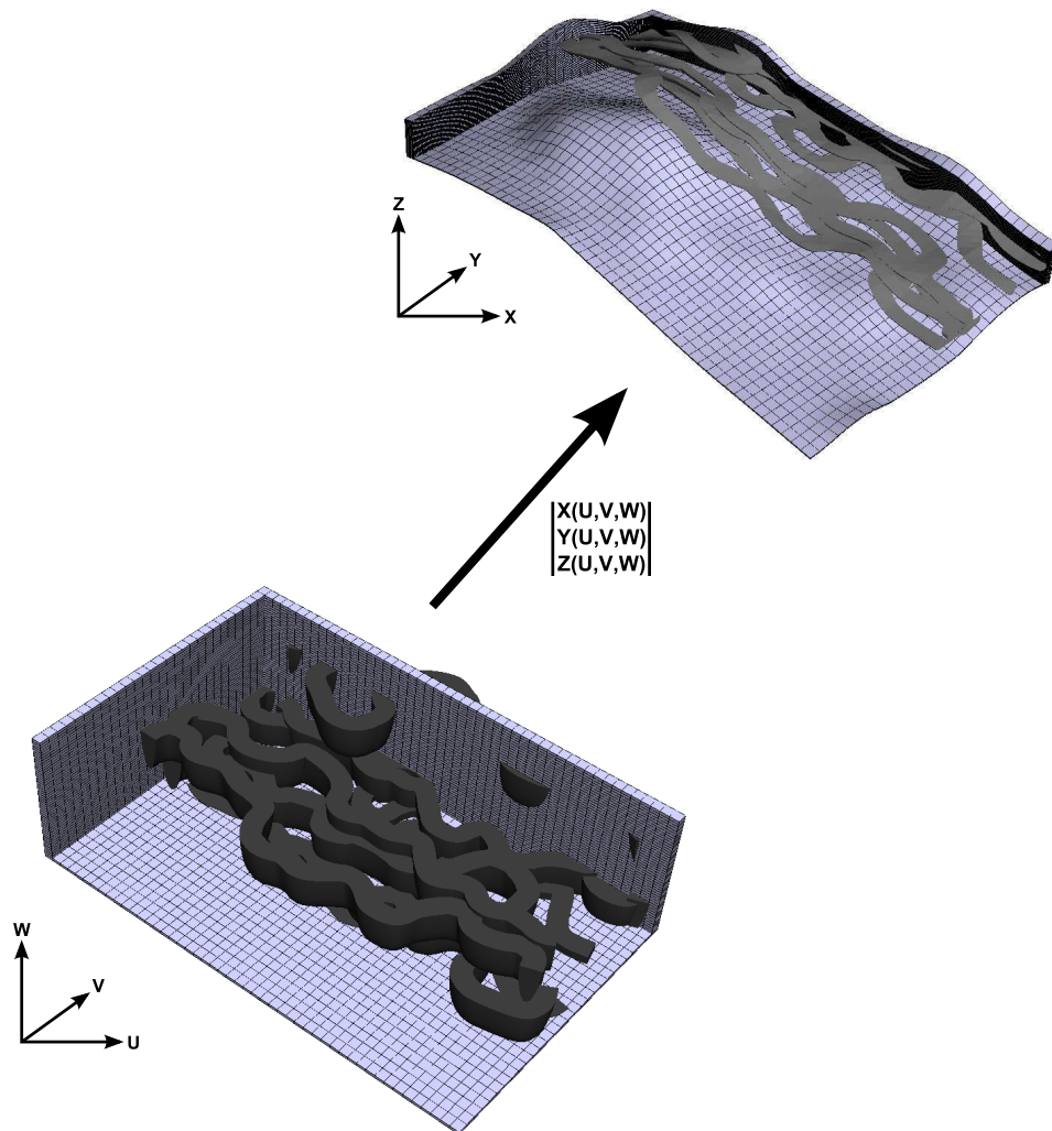
FIGURE 2.25 – MODÈLES DE CHENAUX PLISSÉS. Les chenaux sont modélisés à plat dans l'espace paramétrique d'une grille stratigraphique et la transformation des coordonnées UVW vers XYZ permet de restituer la géométrie déformée des chenaux.
