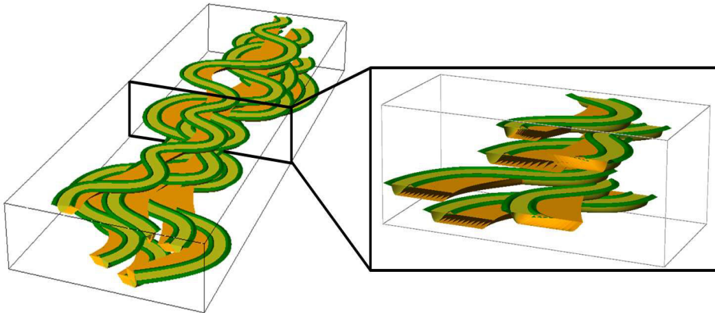
FIGURE 3.13 – RÉALISATION D’UN ENVIRONNEMENT DE DÉPÔT FLUVIATILE PRÉSENTANT QUATRE CHENAUX (EN JAUNE) AVEC LEURS BARRES D’ACCRÉTION LATÉRALE (EN ORANGE) ET LEURS LEVÉES (EN VERT).
