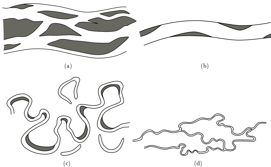
FIGURE 1.2 – DIFFÉRENTS STYLES DE CHENAU, MODIFIÉ D'APRÈS [MIALL, 1977]. (a) Chenaux en tresses avec ces barres fluviales. (b) Chenal droit et ses barres sableuses. (c) Chenal méandrique et ses barres d'accrétion latérale (d) Chenaux anastomosés.
