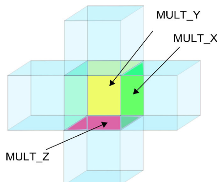
FIGURE 3.25 – LOCALISATION DES MULTIPLICATEURS DE TRANSMISSIBILITÉ COMME DÉFINIS DANS LE SIMULATEUR D'ÉCOULEMENT ECLIPSE, POUR UNE CELLULE IJK.
