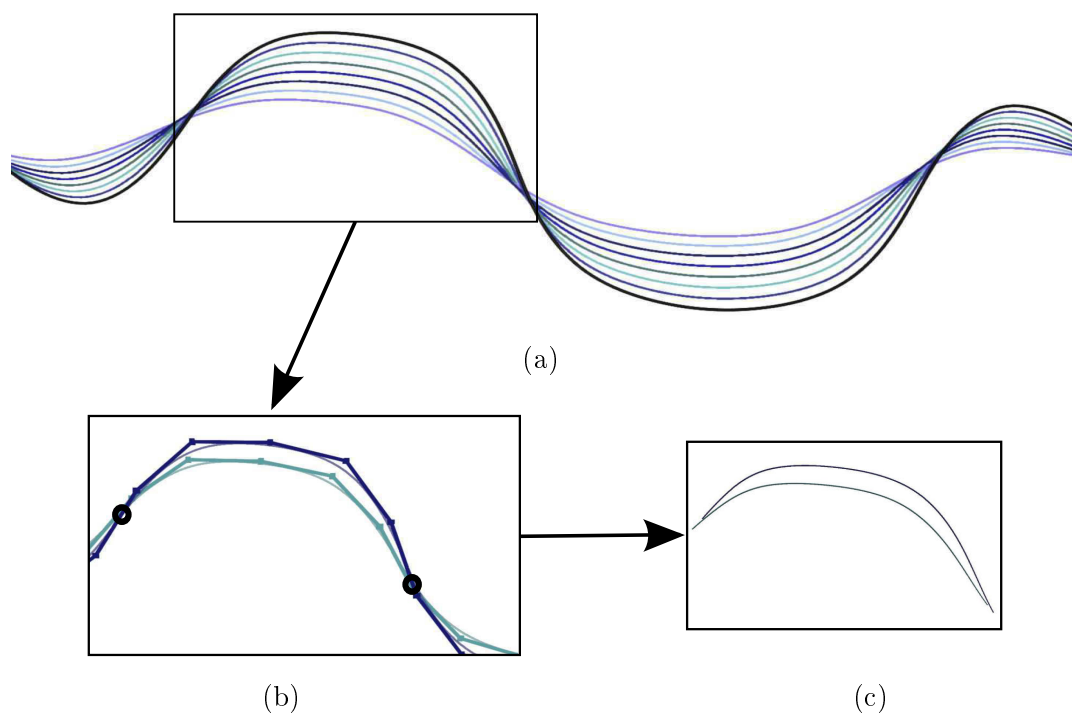
FIGURE 3.11 – EXTRACTION DES CLINOFORMES DES BARRES D'ACCÉTION LATÉRALE À PARTIR DE LA CROISSANCE D'UN CHENAL. Les chenaux sont ici représentés par leurs axes. (a) Un chenal avec ses étapes de croissances. (b) Les intersections entre les maillages de contrôle sont calculés. (c) Portions de chenaux entre les points d'intersections.
