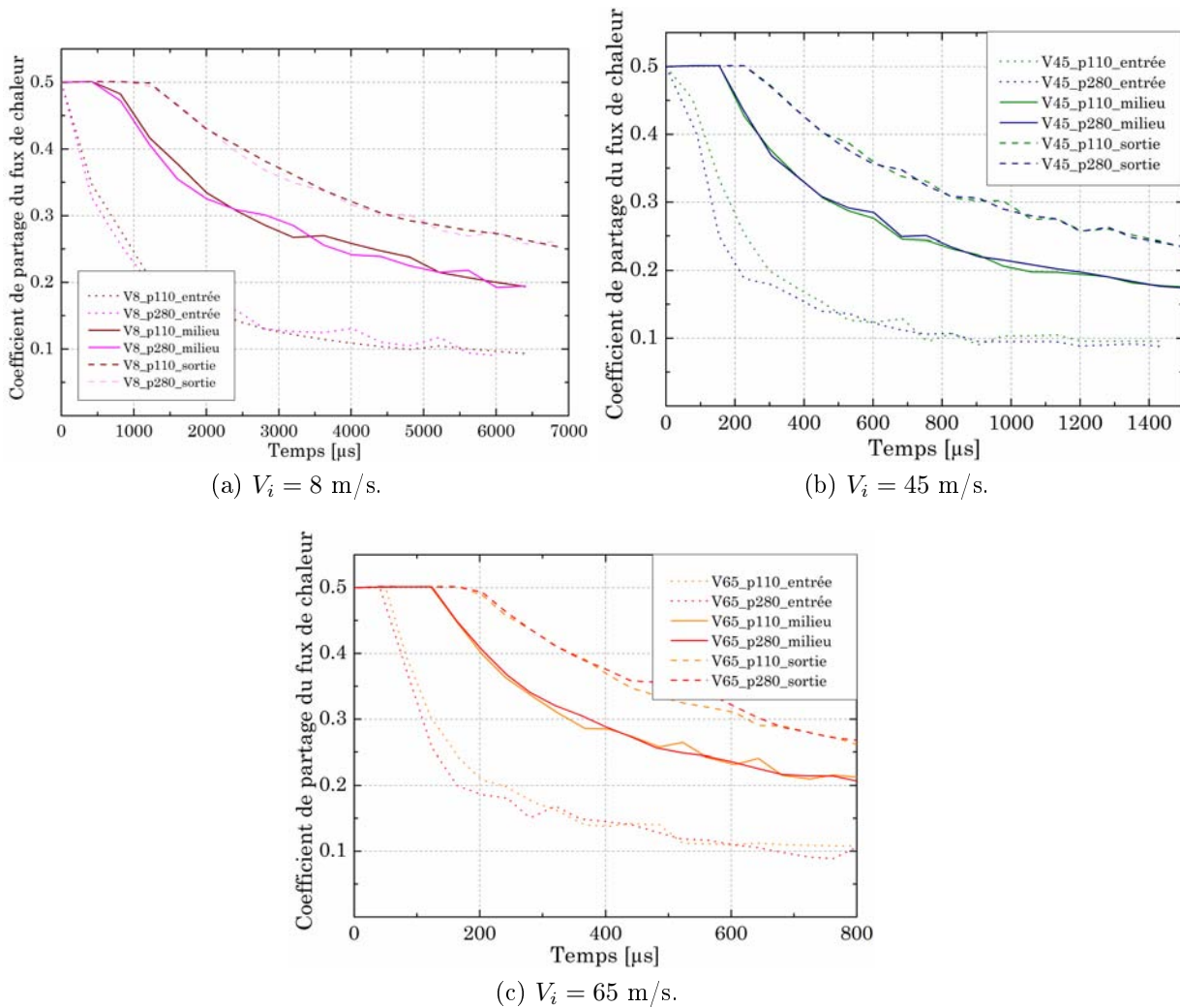
FIGURE 3.13 – Coefficients de partage locaux du flux de chaleur en fonction du temps de glissement.
