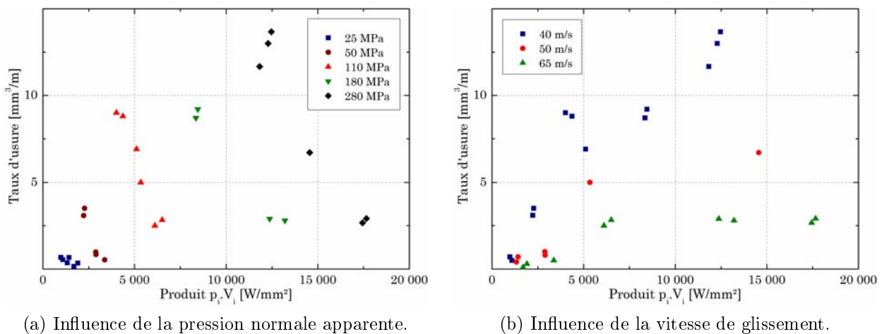
FIGURE 4.10 – Évolution du taux d'usure en fonction du produit p_i \cdot V_i .
