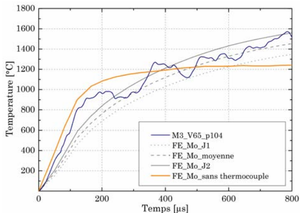
(d) V_i = 65 \text{ m/s } p = 110 \text{ MPa} .
