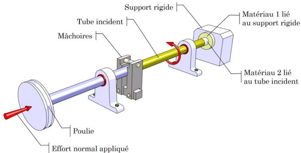
FIGURE 2.2 – Principe de fonctionnement des barres de Kolsky modifiées pour mesurer le coefficient de frottement \mu .
