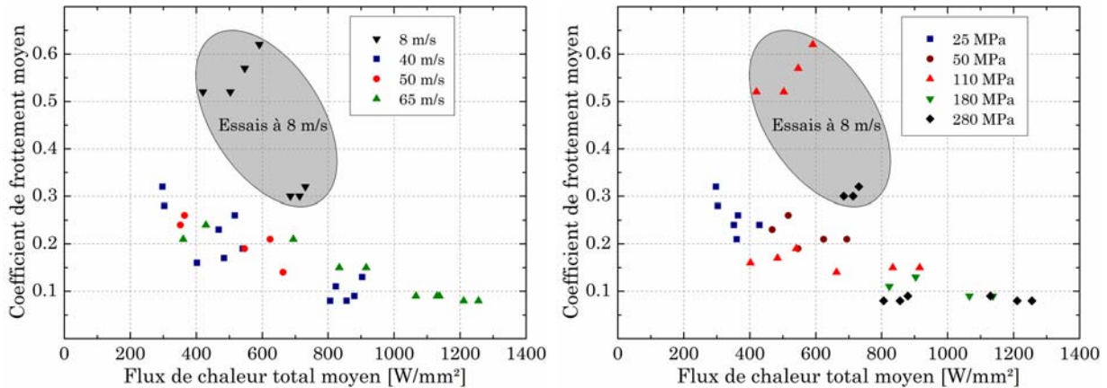
(a) En fonction de la vitesse initiale de glissement V_i . (b) En fonction de la pression normale apparente initiale p_i .
