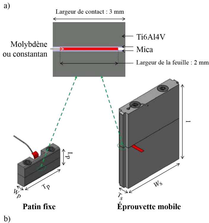
Figure 2.18 – Intégration du thermocouple feuille-pièce au sein des pièces en Ti6Al4V.
