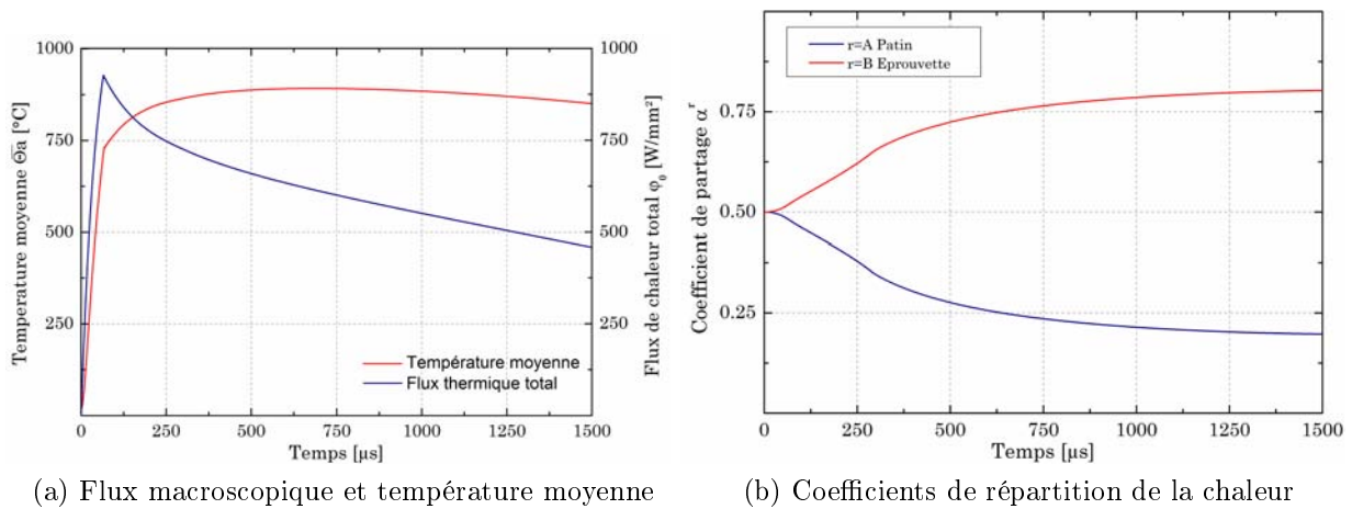
FIGURE 5.11 – Résultats issus du modèle semi-analytique - Grandeurs thermiques macroscopiques (essai à V_i = 40 m/s, p = 100 MPa et f = 6 %)
