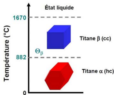
FIGURE 1.7 – Cristallographie du titane pur [Gautier 2004].
