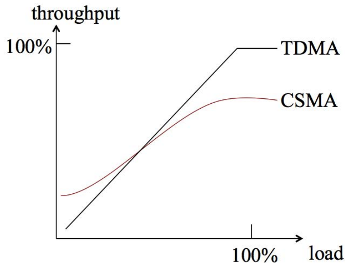
FIGURE 3.14 – Comparaison de l'efficacité entre méthodes basées sur la contention (CSMA) et sur l'ordonnancement (TDMA) en fonction du débit réseau. (Source : [Song, 2013])
