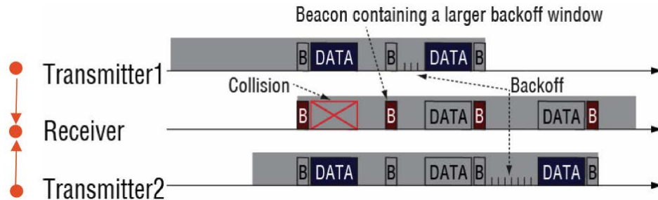
FIGURE 3.12 – Illustration de la méthode BEB (Binary Exponential Backoff) employée par RI-MAC pour résoudre les problèmes de collisions dus à l’envoi simultané de trames par plusieurs émetteurs. (Source : [Song, 2013] d’après [Sun et al., 2008])
