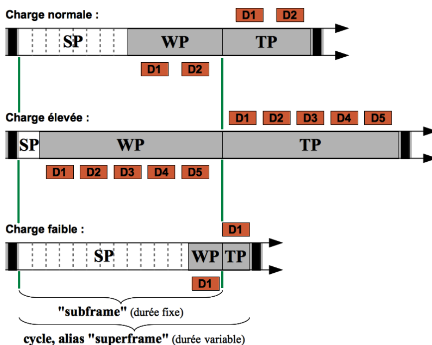
FIGURE 3.16 – Principe d'un cycle de fonctionnement d'un noeud coordinateur S-CoSenS. (D'après [Nefzi, 2011])
