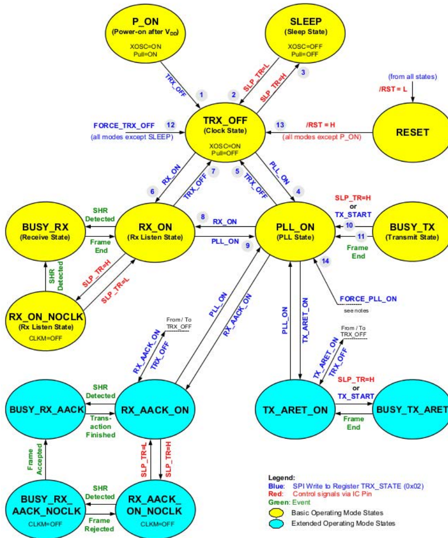
FIGURE 6.2 – Diagramme complet de la machine à états finis de l'AT86RF231. (Source : [DataSheet AT86RF231, 2009] figure 7-8.)
