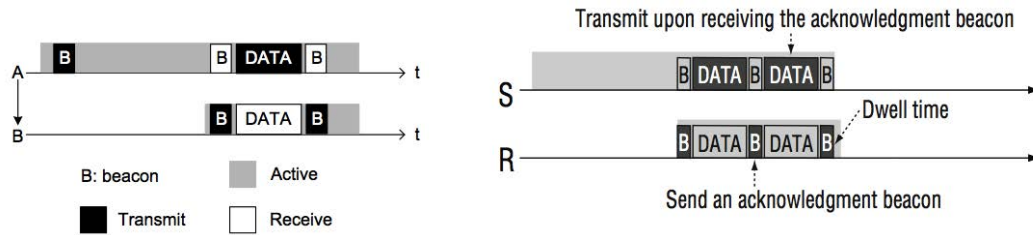
FIGURE 3.11 – Principe de transmission de données entre un noeud émetteur ( A ou S ) et un noeud récepteur ( B ou R ), selon la méthode RI-LPP (Receiver-Initiated Low Power Probing). (Source : [Song, 2013] et [Huang et al., 2013])
