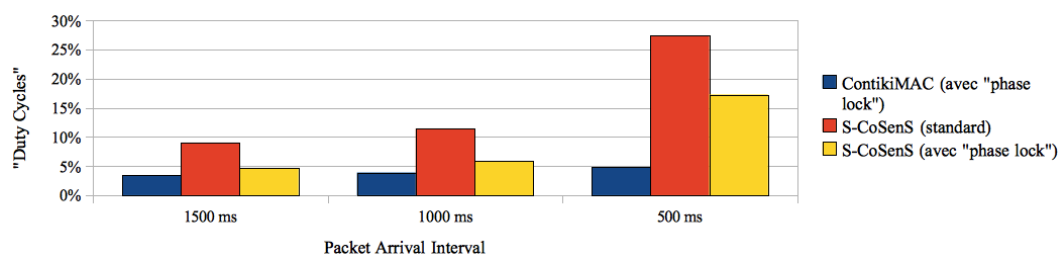
FIGURE 5.19 – Influence du mécanisme de “ phase lock ” sur l’activité radio ( duty cycle ) induite par S-CoSenS et ContikiMAC, avec respectivement des subframes de 125 ms et des CCI de 8 Hz.
