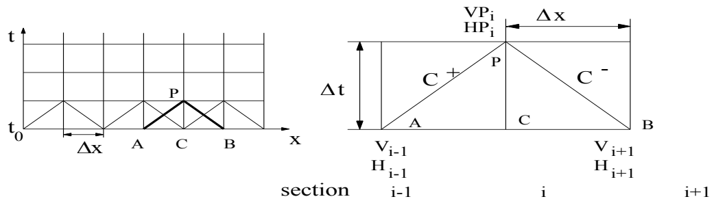
Figure II-18. Calcul du coup de bélier par la méthode des caractéristiques
