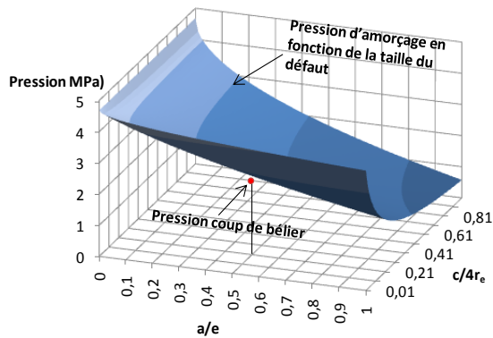
Figure V-14. Représentation tridimensionnelle de la pression d'amorçage en fonction de la taille du défaut
