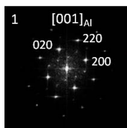
(b) Zone GP-I parallèle au plan (010)_{Al}
