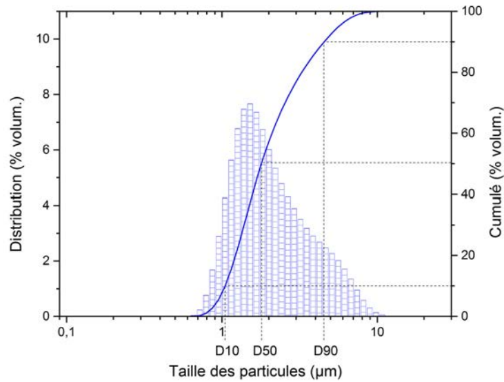
FIGURE IV.1 – Distribution granulométrique de la poudre de B 4 C déterminée avec un granulomètre Laser.
