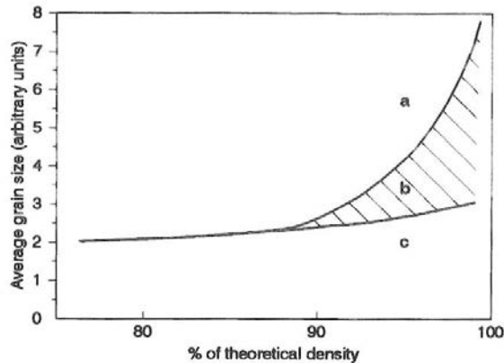
FIGURE I.19 – Dépendance de la taille moyenne des grains sur la densité du fritté (schéma) (a) sans ajout d’inhibiteur à la croissance des grains, (b) avec inhibition partielle, (c) avec une forte inhibition à la croissance des grains (extrait de [90]).
