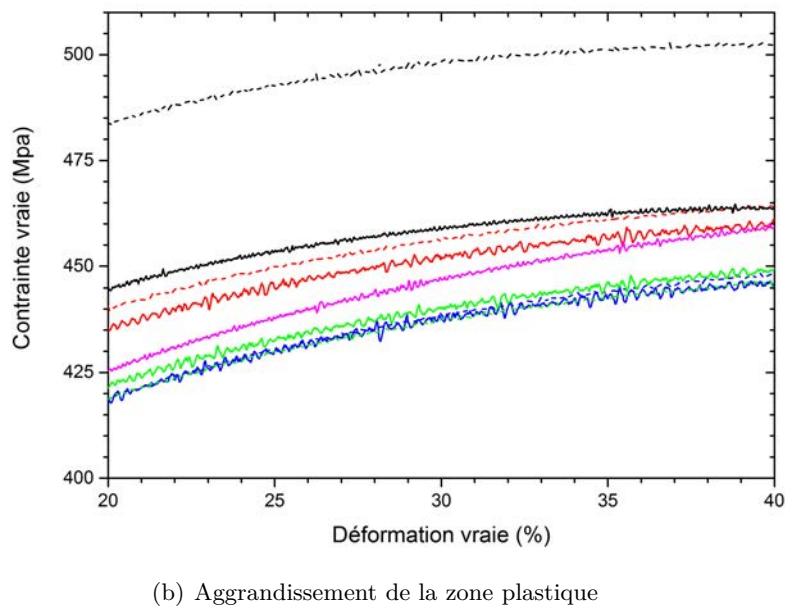
FIGURE IV.7 – Courbes contrainte vraie-déformation vraie en condition de compression quasistatique à 10^{-3} s^{-1} des composites issus de mélange.
