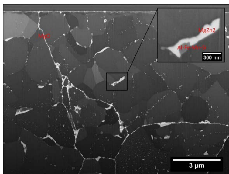
FIGURE II.10 – Micrographie MEB en électrons secondaires du lot A brut consolidé après découpe par FIB.
