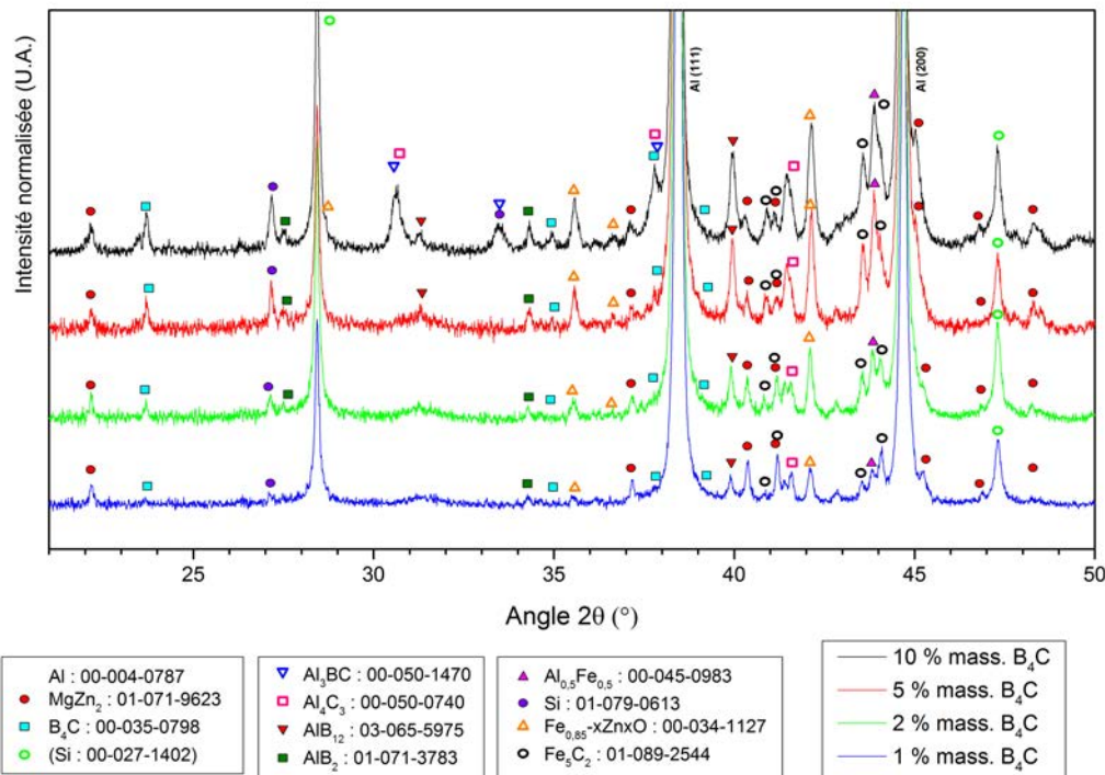
FIGURE IV.15 – Diffractogrammes de rayons-X des composites chargés à 1, 2, 5 et 10 % mass. B_4C issus du broyage consolidés à 500\text{ }^\circ\text{C} sous 80 MPa avec un maintien de 10 minutes ( \lambda = 0,154\text{ nm} ).
