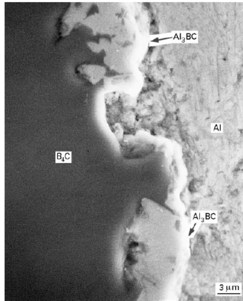
FIGURE I.9 – Vue MEB détaillée de l'interface Al– \text{B}_4\text{C} après 15 h de réaction à 1000 K (extrait de [70]).
