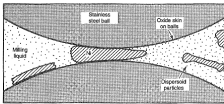
(a) État initial : le nickel est aplati en formes de pétales ; les renforts s'incrustent dans les particules.
