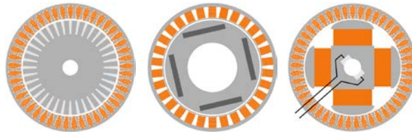
Figure: Technologie de machines électriques utilisées dans les véhicules hybrides ou électriques
