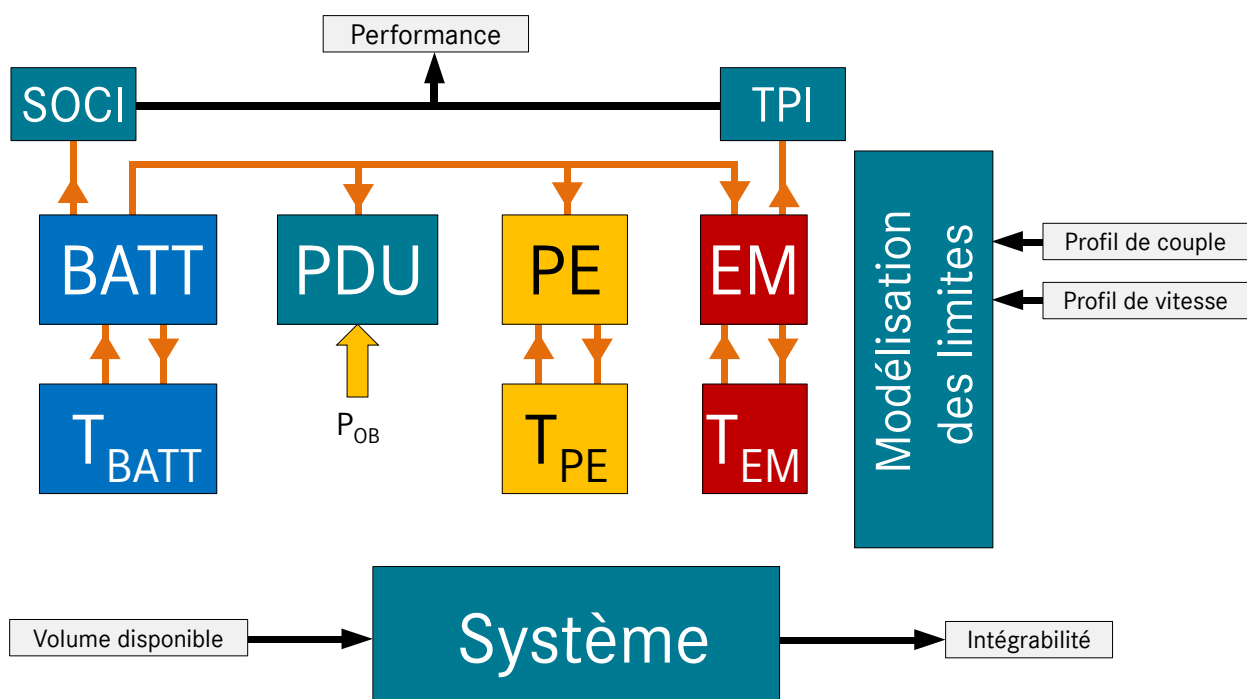
Figure: Implémentation du modèle global du système électrique
