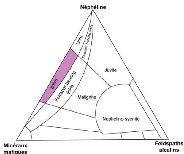
FIGURE 2.8 – Diagramme ternaire de classification des minéraux mafiques - néphéline - feldspaths alcalins, modifié à partir de Elías-Herrera et al. (1991)
