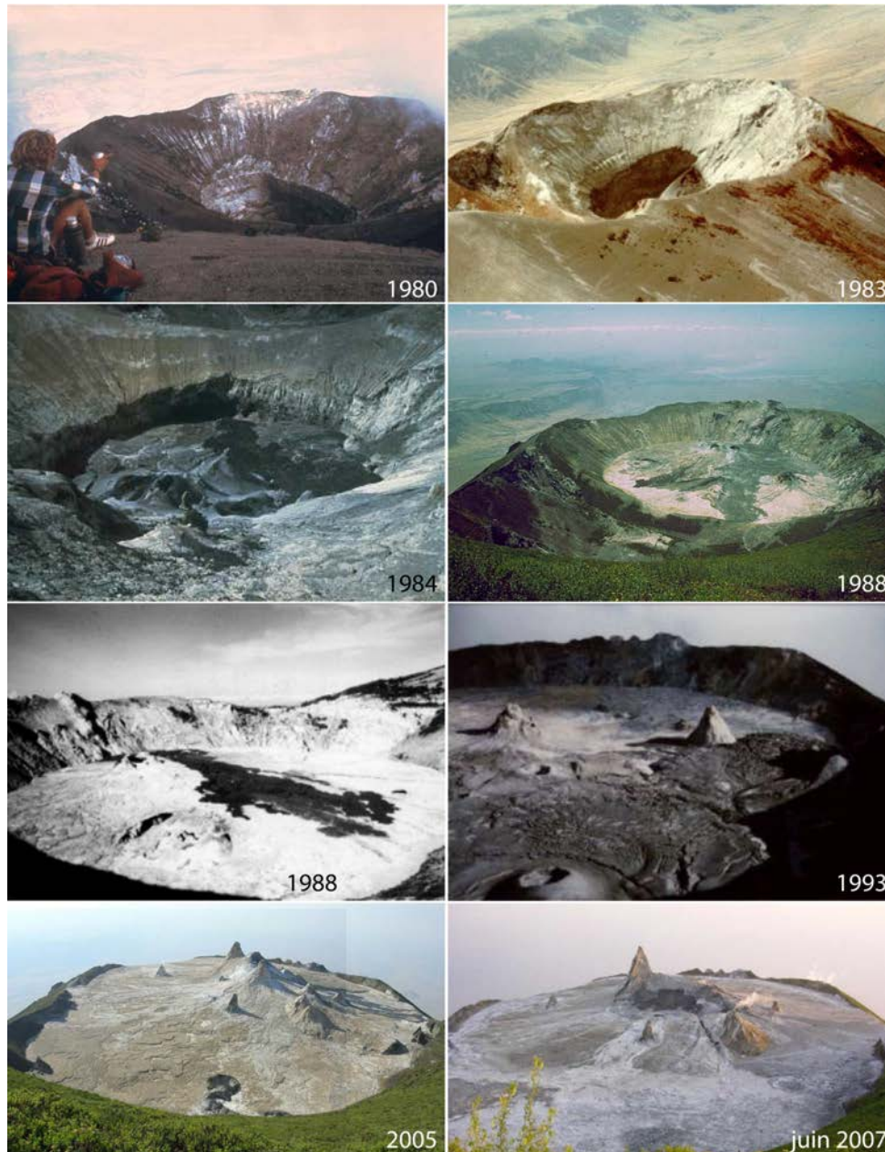
FIGURE 1.17 – Photographies de l’Oldoinyo Lengai de 1967 à 1988.
