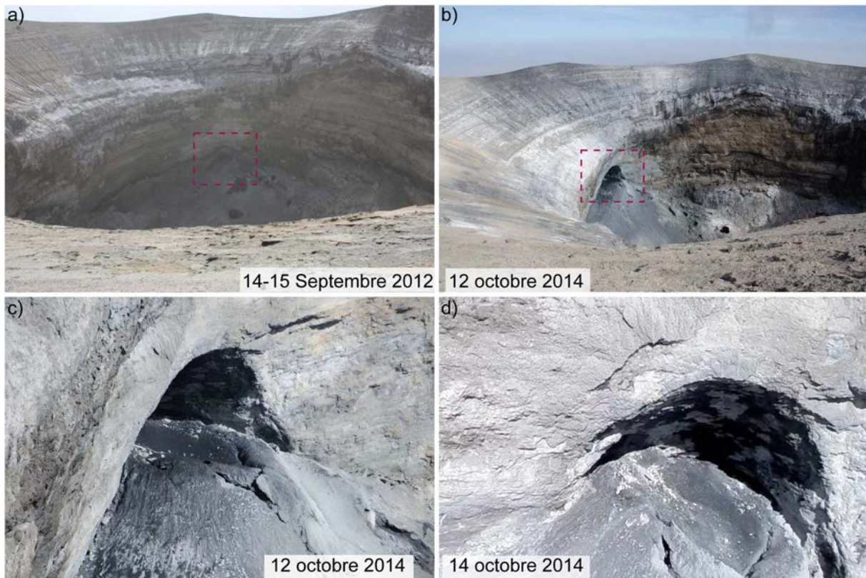
FIGURE 2.3 – a) Vue d’ensemble du cratère le 14-15 septembre 2012. (Source : Frank Möckel et Wendy Blank, volcano.si.edu) Photographies de l’intérieur du cratère nord en 2014 : b) Vue d’ensemble prise le 12 octobre 2014. Zoom à l’intérieur du cadre rouge en pointillé de la photographie (b) : c) le 12 octobre 2014 et d) le 14 octobre. Entre 2013 et 2014, l’hornito sur la paroi ouest du cratère nord a pris de l’ampleur. Entre le 12 et 14 octobre la lave au sommet de celui-ci s’est blanchie, caractéristique de l’altération des natrocarbonatites.
