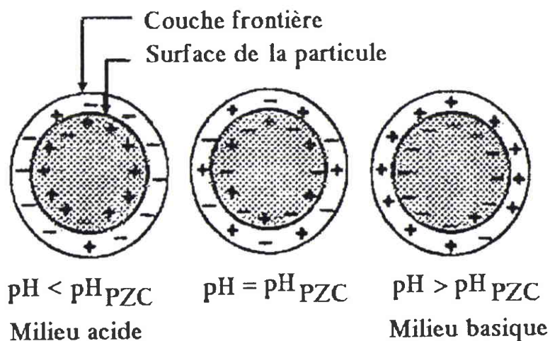
Figure 4. 2 : Accessibilité chimique du précurseur métallique en fonction du pH de la solution
