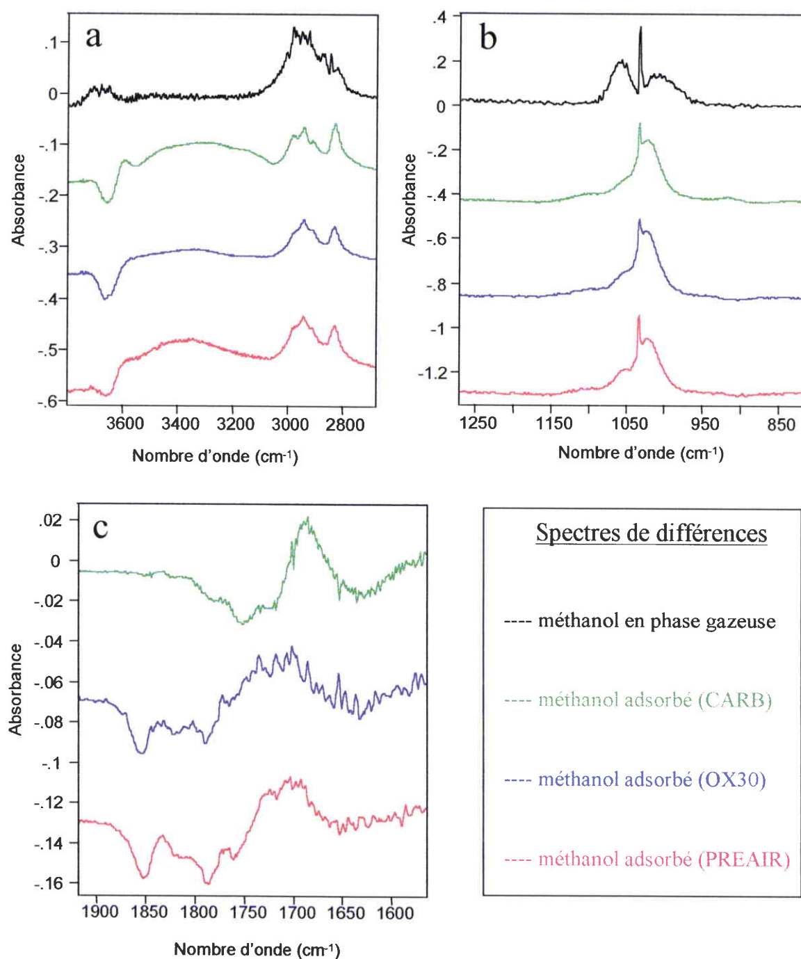
Figure 4. 6 : Spectres du méthanol adsorbé sur différents supports carbonés. Régions analytiques : a) 3700\text{-}2700\text{ cm}^{-1} ; b) 1270\text{-}810\text{ cm}^{-1} et c) 1930\text{-}1550\text{ cm}^{-1} .
