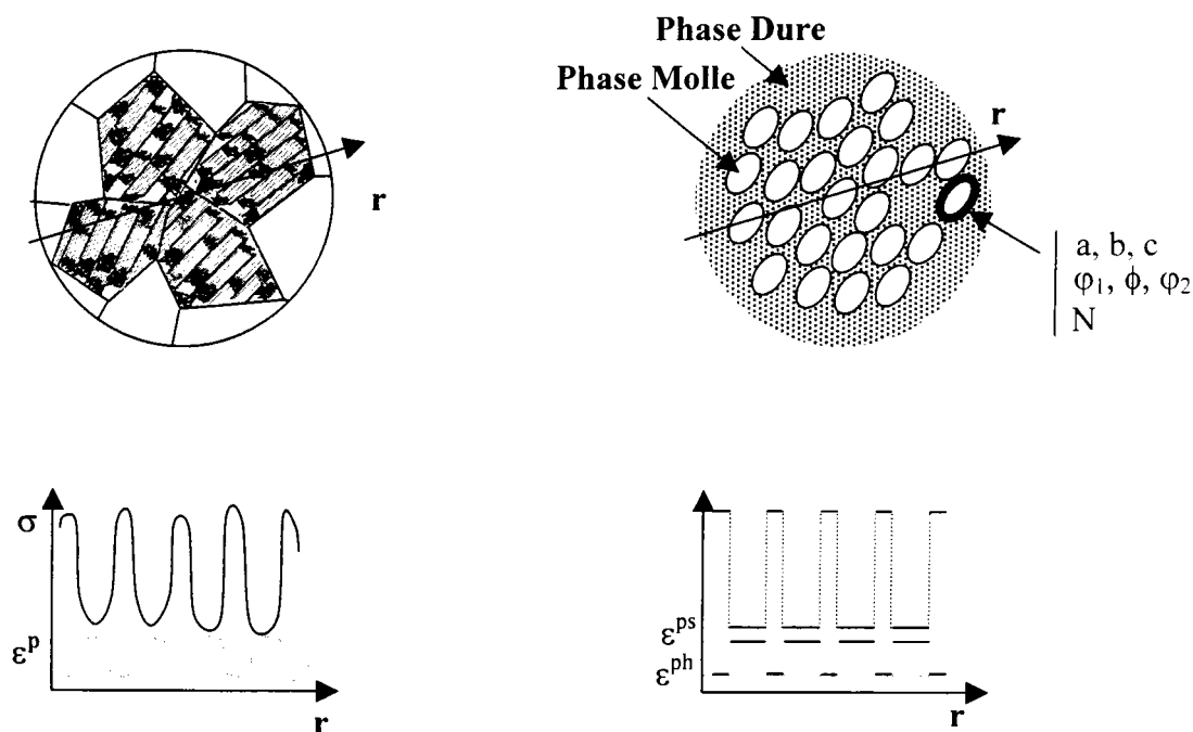
Figure II.2 : représentation de la microstructure de dislocation par un matériau biphase à structure évolutive et écoulement non local
