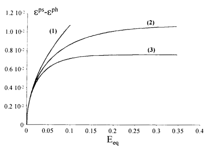
Figure III.7d: saut de déformation plastique équivalente
