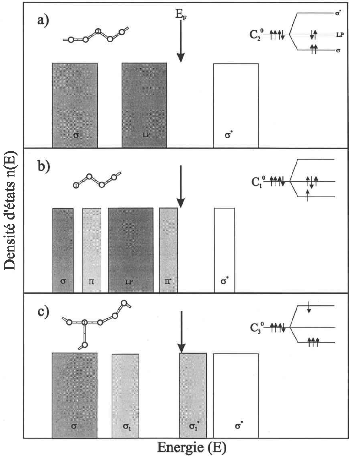
Figure V.18 : Représentation schématique de la densité d'états n(E) 4 pour : a) une structure en chaînes C_2^0 , b) un centre C_1^0 avec l'apparition des pics \pi et \pi^* dû à une liaison \pi avec l'atome voisin, c) un centre C_3^0 où 1 électron occupe une orbitale antiliante \sigma_1^* .
