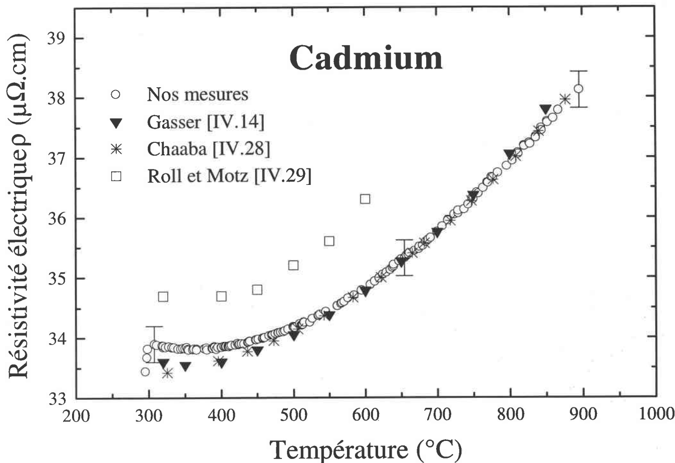
Figure IV.9 : Résistivité électrique du cadmium liquide en fonction de la température.
