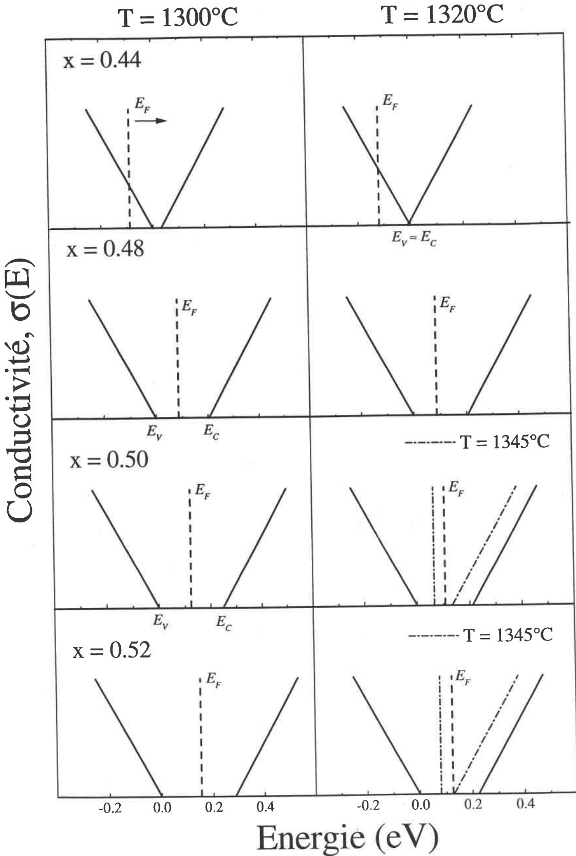
Figure V.21 : Représentation de \sigma(E) pour l'alliage liquide \text{Zn}_x\text{Te}_{1-x} à différentes températures. La largeur du gap \Delta E_G et la position de l'énergie de Fermi E_F sont déduites de la figure V.19.
