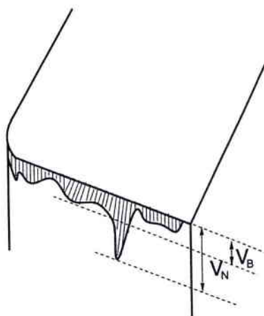
FIG. 2.5 - Usure en entaille.
