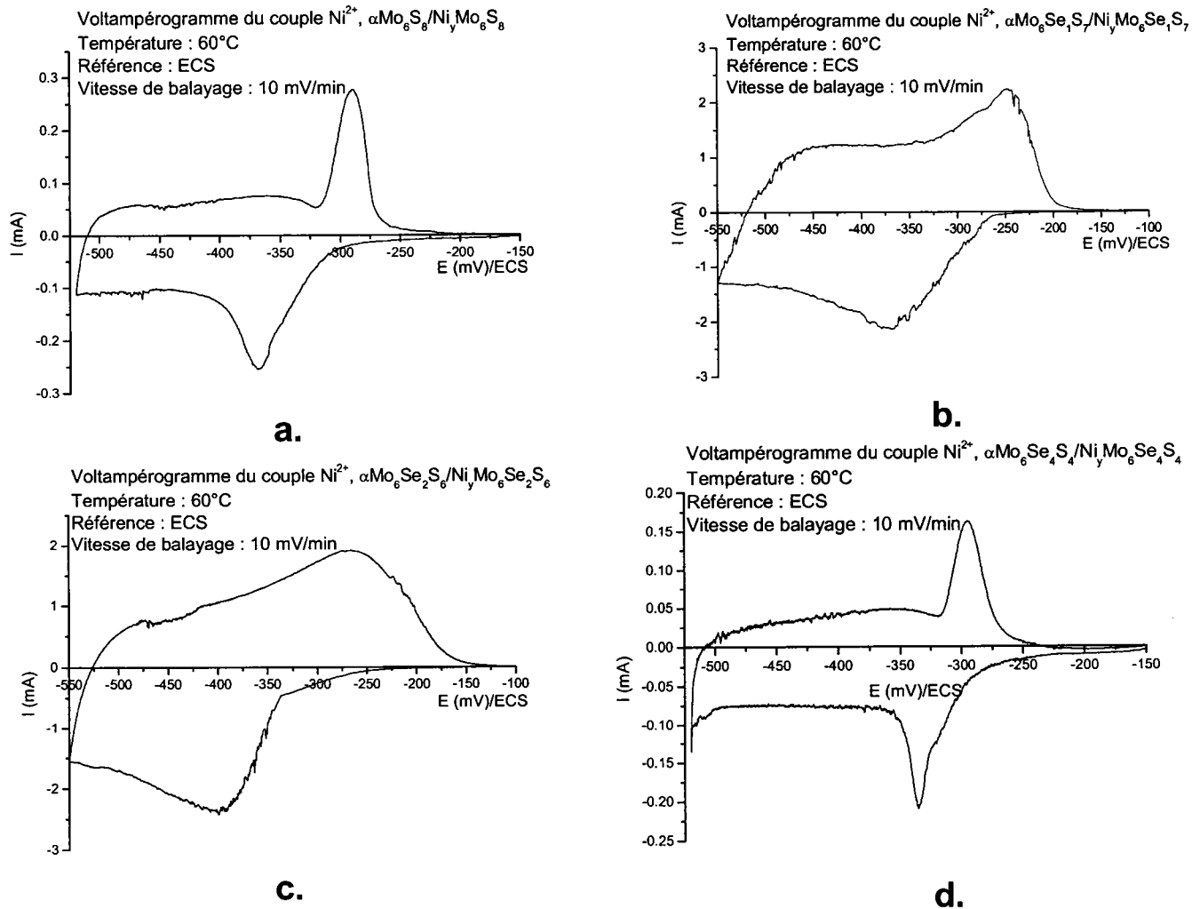
Figure III.4.4 : Voltampérogrammes des systèmes \text{Ni}^{2+} , \alpha\text{Mo}_6\text{Se}_{8-x}\text{S}_x/\text{Ni}_y\text{Mo}_6\text{Se}_{8-x}\text{S}_x (vitesse de balayage : 10mV/min)
