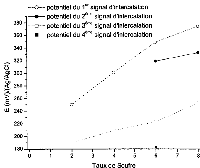
Figure III.3.7 : Evolution des potentiels des signaux d'intercalation de \text{Cu}^{2+} dans les phases \beta\text{Mo}_6\text{Se}_{8-x}\text{S}_x .
