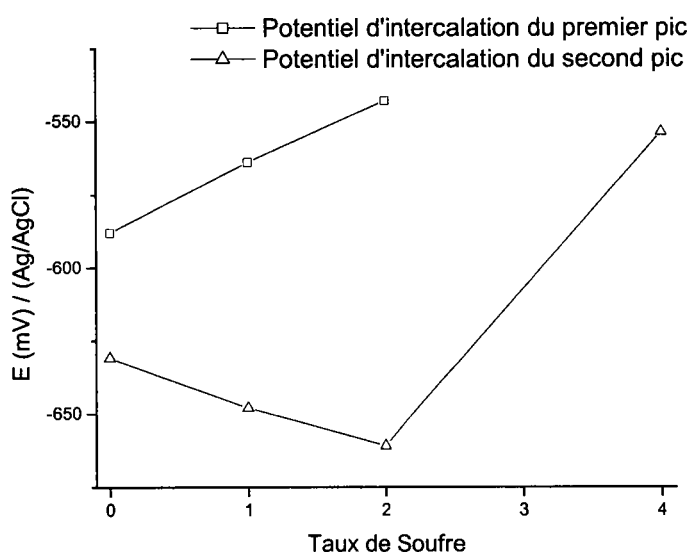
Figure III.1.16 : Evolution des potentiels des signaux d'intercalation de Zn^{2+} dans les phases HTMo_6Se_{8-x}S_x .
