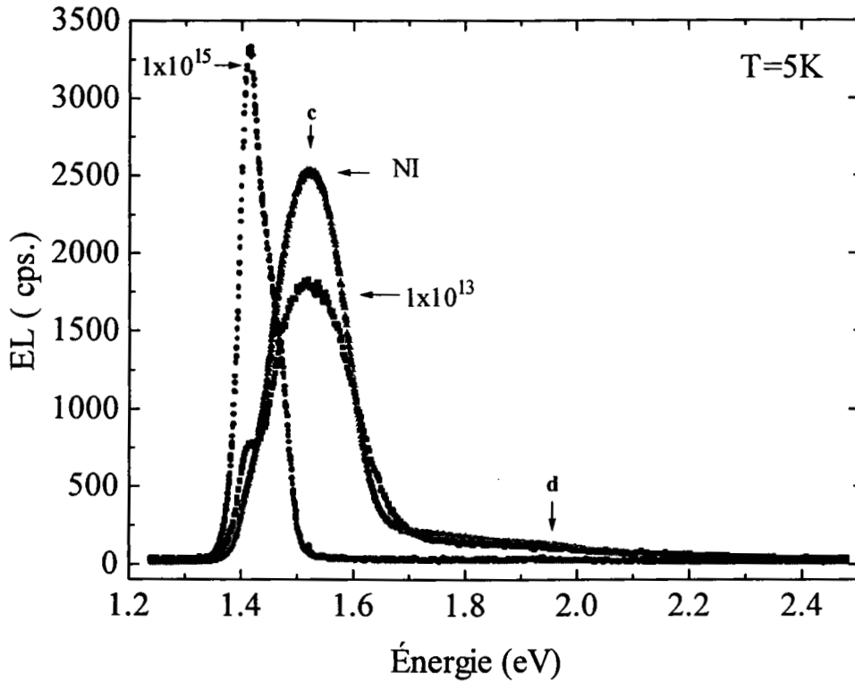
Fig. V-13: Spectres d'EL des jonctions à base de GaAs polarisées en avalanche (10 mA), aux fluences de neutrons : NI et 1 \times 10^{13} et 1 \times 10^{15} n/cm 2 .
