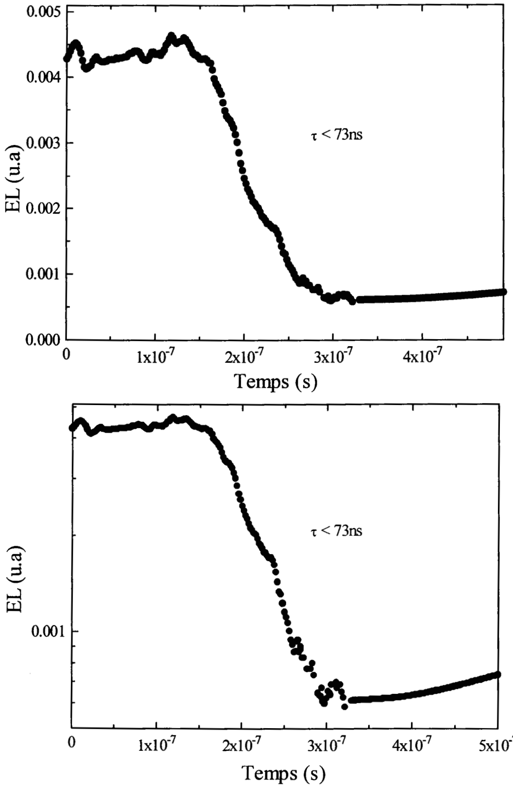
Fig. VI- 3: Signal d'EL résolue en le temps de la jonction E-B des transistors bipolaires (NPN) à base de Si polarisée en avalanche. La courbe inférieure est en échelle logarithmique.
