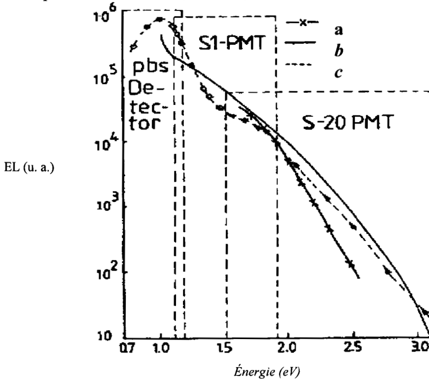
Fig. IV- 7 : Comparaison de : (a) spectre de Toriumi [43], (b) spectre de Chynoweth et al. [6] et (c) spectre mesuré avec trois détecteurs différents: PbS, S1 et S-20 [9].
