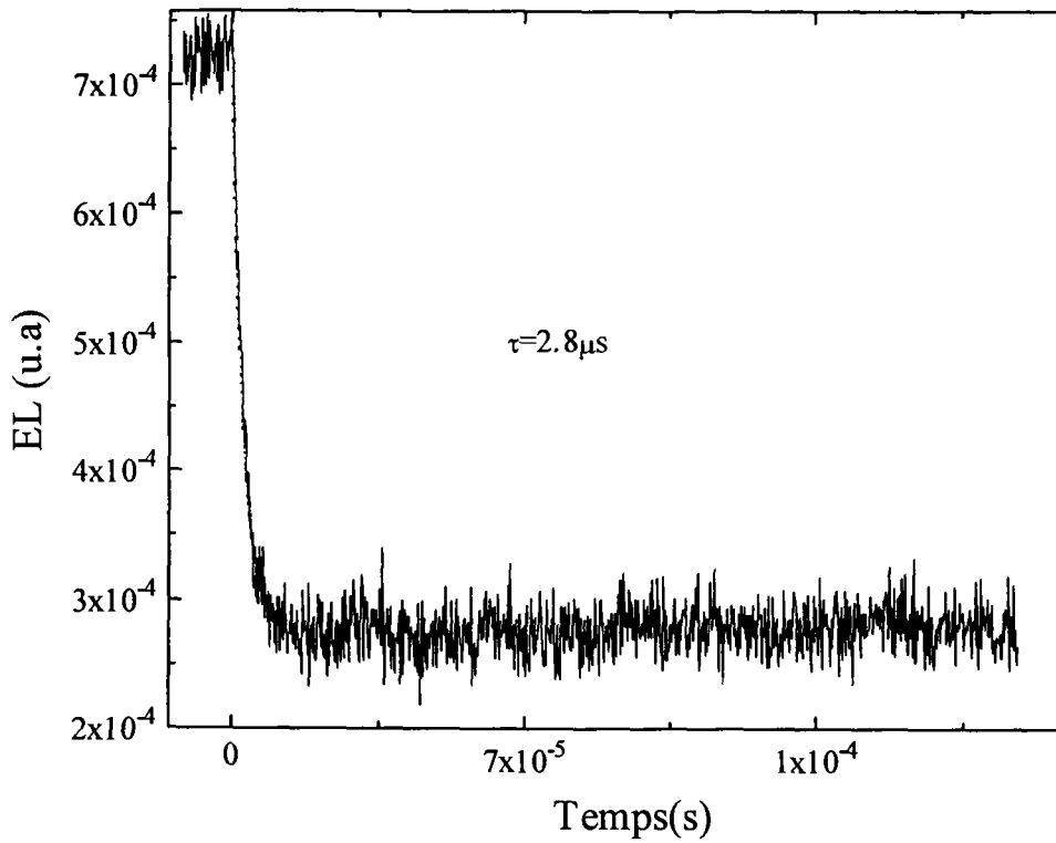
Fig. VI- 1: Signal d'EL résolue en temps de la jonction E-B des transistors bipolaires (NPN) à base de Si polarisée en direct. Représentation en échelle linéaire.
