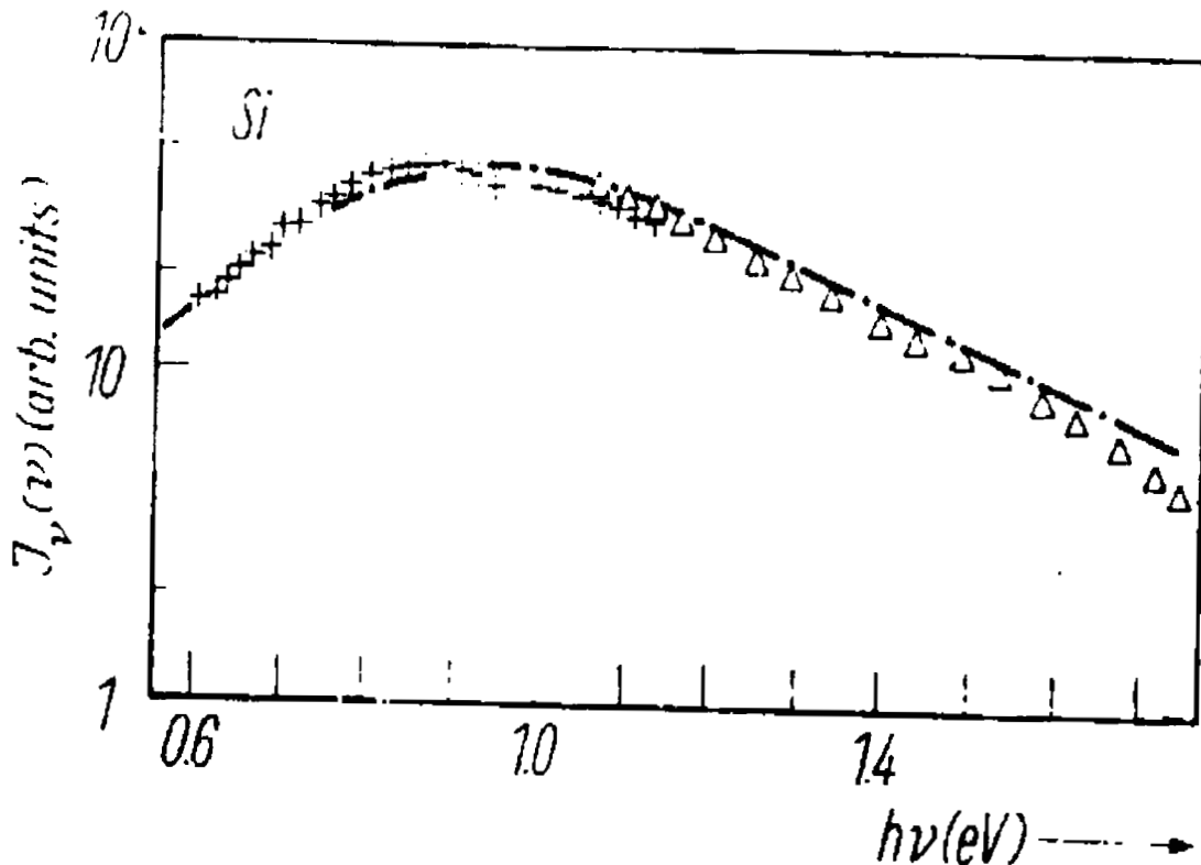
Fig. IV- 33 : Comparaison de la radiation expérimentale donnée par le Si (+) pour des énergies inférieures à l'énergie du gap; (( \Delta ) Chynoweth, McKay, (- . - . -) est le spectre théorique des transitions directes.
