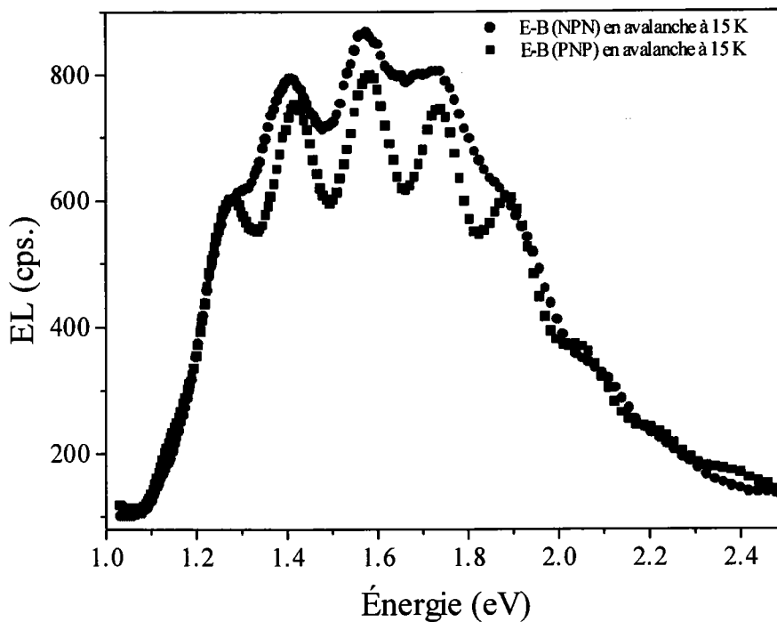
Fig. IV- 26 : Intensité d'EL en fonction de l'énergie du photon pour les jonctions E-B (NPN et PNP) polarisées en avalanche, à la température de 15 K.
