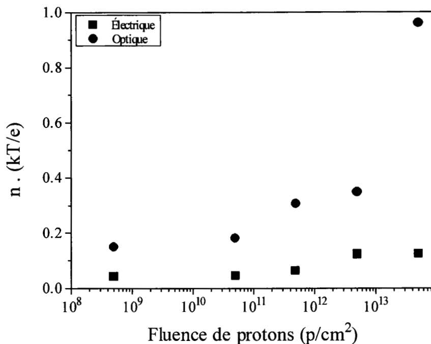
Fig. III- 11: L'évolution de la quantité n(kT/e) électrique et optique en fonction de la fluence de protons pour I(V) et EL(V) des jonctions E-B des transistors bipolaires PNP polarisées dans le mode direct.
