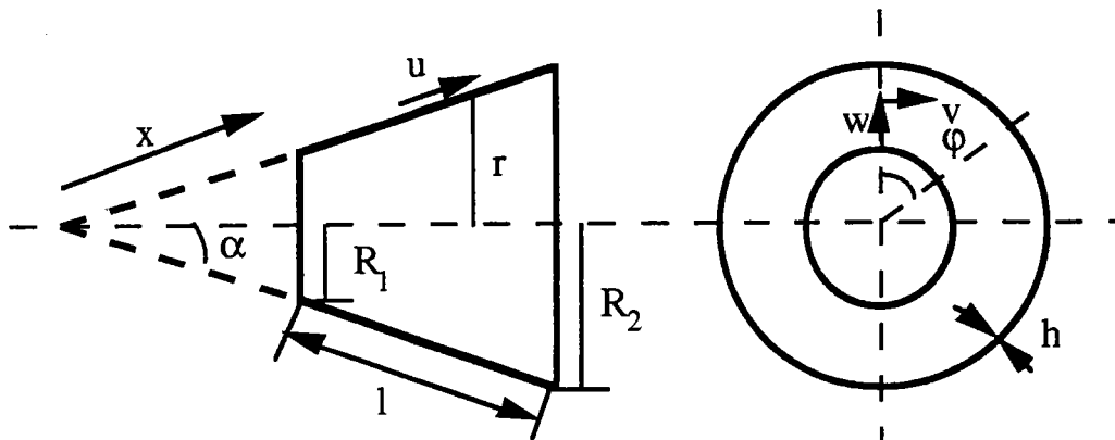
fig. V-3 Géométrie de la coque tronconique
