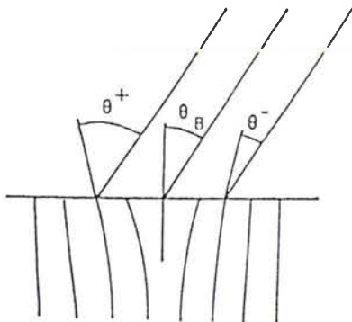
Fig. 12. — Le contraste du grain A s'inverse pour une rotation de 90° de l'échantillon.
