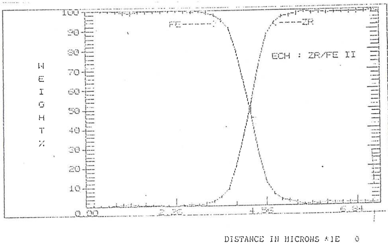
figure 77 : Profil de concentration du couple Zr CL / Acier (650°C - 600 daN - 8h 48 mn).
