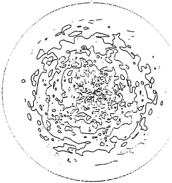
a- figure de pôle (101)
