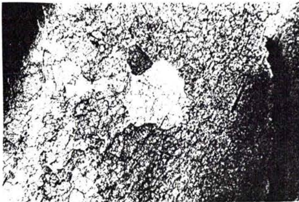
c- G= 50 formation de sous grains couple Zy pc / Al / Zérodure.
