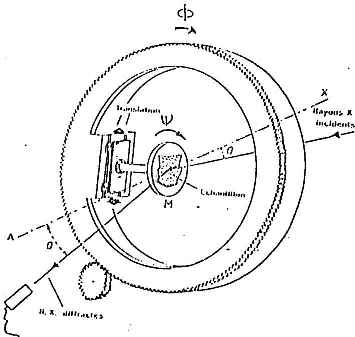
Fig. (6) : Principe du goniomètre de texture
