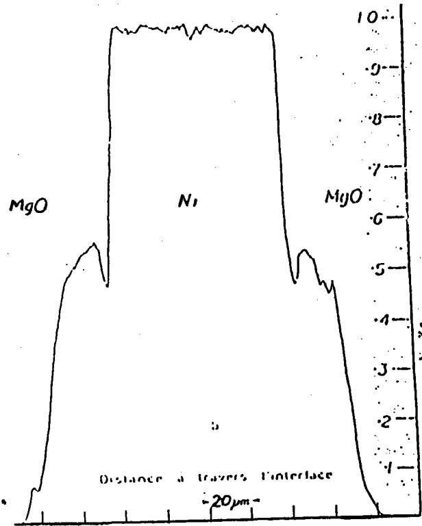
Répartition du Ni (trace K\alpha du Ni) 1100°C - 16 heures dans l'air figure 9 : interface céramique-métal présence d'une 3 ème phase./38/
