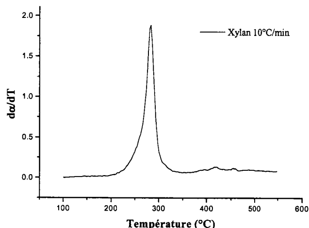
Figure II.17 : Courbe dérivée de la perte de masse pour la pyrolyse du xylan à 10°C.min -1
