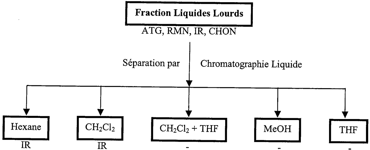
Figure III.20 : Méthodes de caractérisation des liquides lourds utilisées
