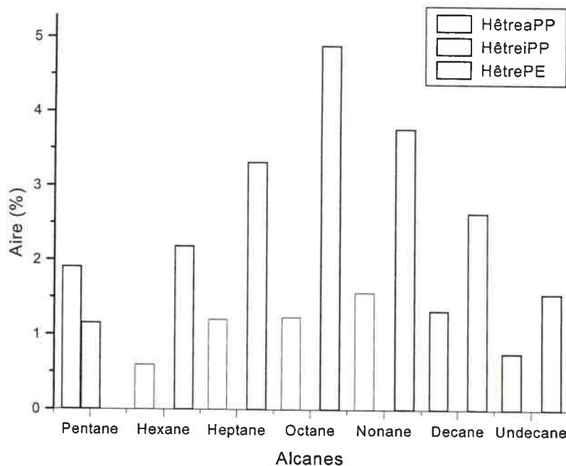
Figure III.14 : Proportions d’alcane non-substitués entrant dans la composition des liquides légers issus de la co-pyrolyse hêtre-plastique (aPP, iPP et PE)
