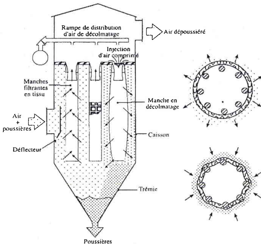
Figure 7 : Filtre à manches [24]
