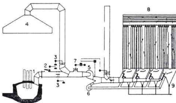
Figure 6 : Système d'aspiration des fumées [17]
