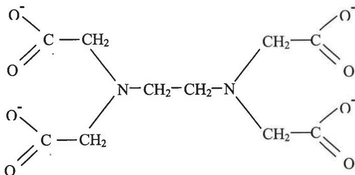
l'anion éthylènediaminetétraacétate
