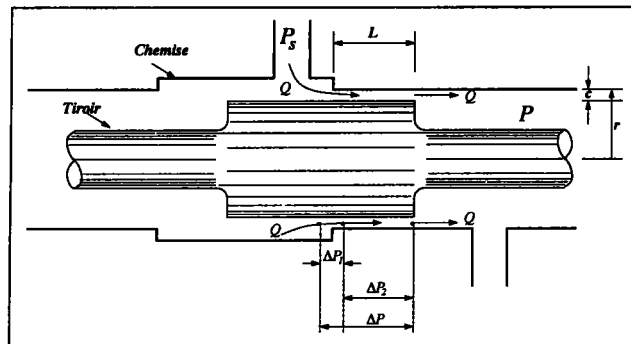
FIG. 0.1 – Tiroir-chemise en position de recouvrement
