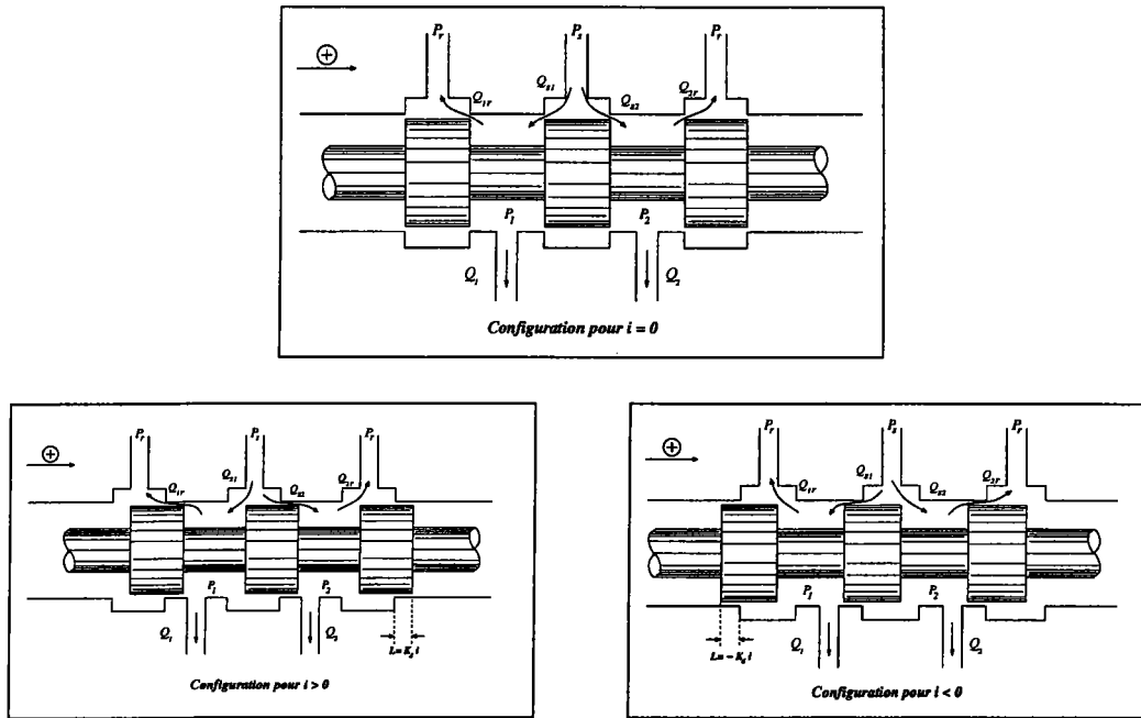
FIG. 0.3 – Configuration d'un tiroir à centre critique
