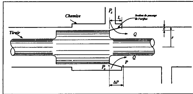
FIG. 0.2 – Tiroir-chemise en position de découverture
