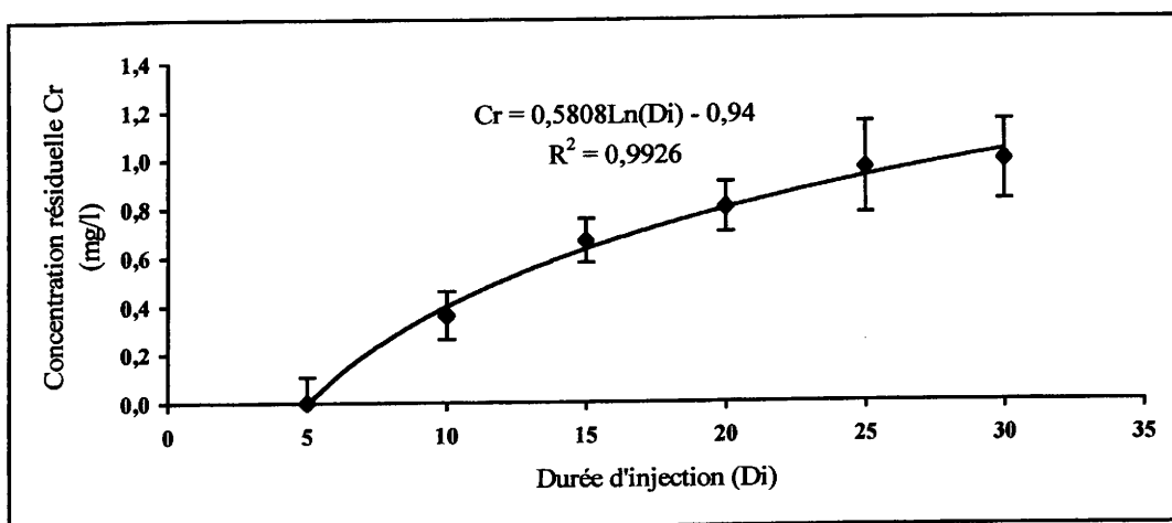
Figure V.4. : Evolution de la concentration de Mexel® 432 dans le bac exposé n° 3 durant 30 minutes.
