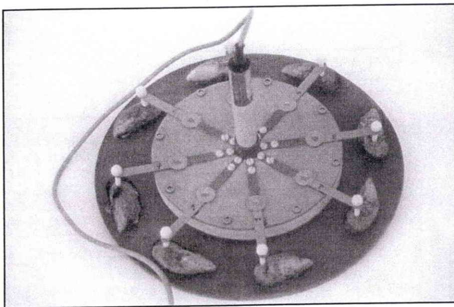
Figure I.6. : Photographie du 'Valvomètre' (IFREMER-Micrel).
