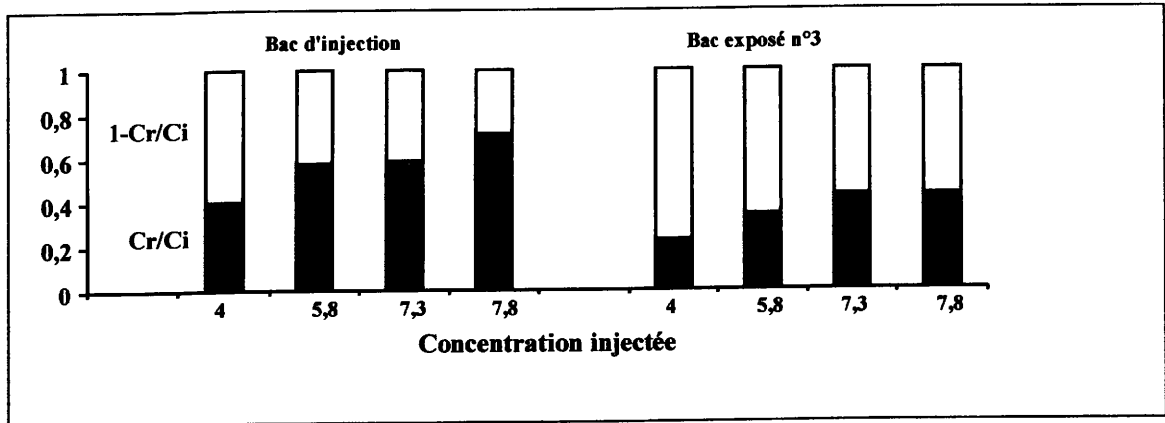
Figure V.3. : Stabilité du Mexel ® 432 dans le bac d'injection et exposé n°3. Cr/Ci : Dégradation du Mexel ® 43, 1-Cr/Ci : Demande de l'eau de Moselle.
