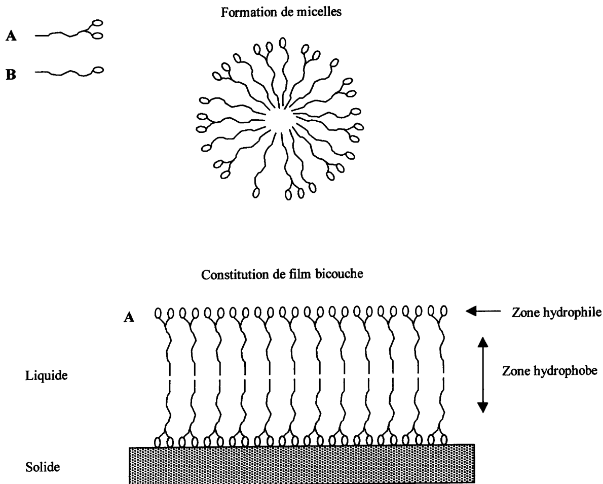
Figure L2. : Représentation schématique des micelles et du film bicouche (d'après Allonier et al. , 1997).
