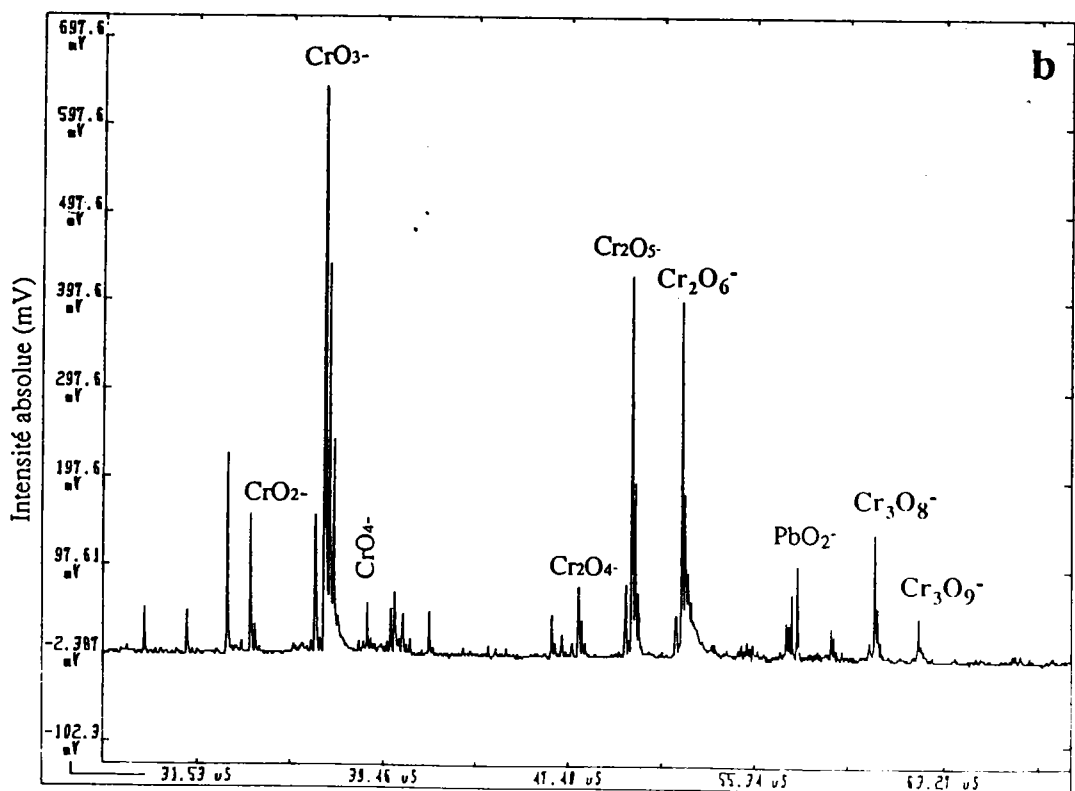
Figure. 24 : Spectre LAMMA en mode négatif de deux types de particules de dérivés chromés ( CrIII 24a et CrVI 24b)
