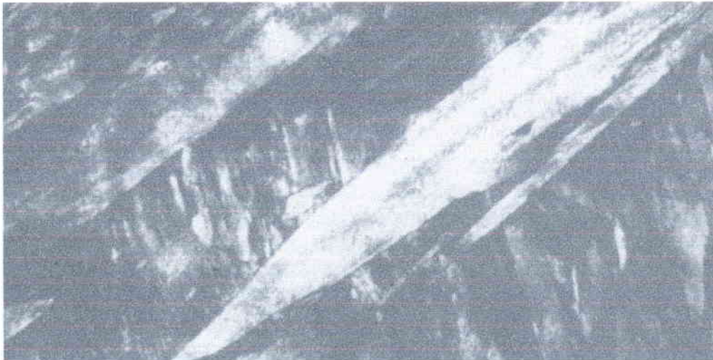
Figure II.5 : Micrographie d'une plaquette de martensite en latte . Observation au MET (alliage FE-0,4%C) [WA90]
