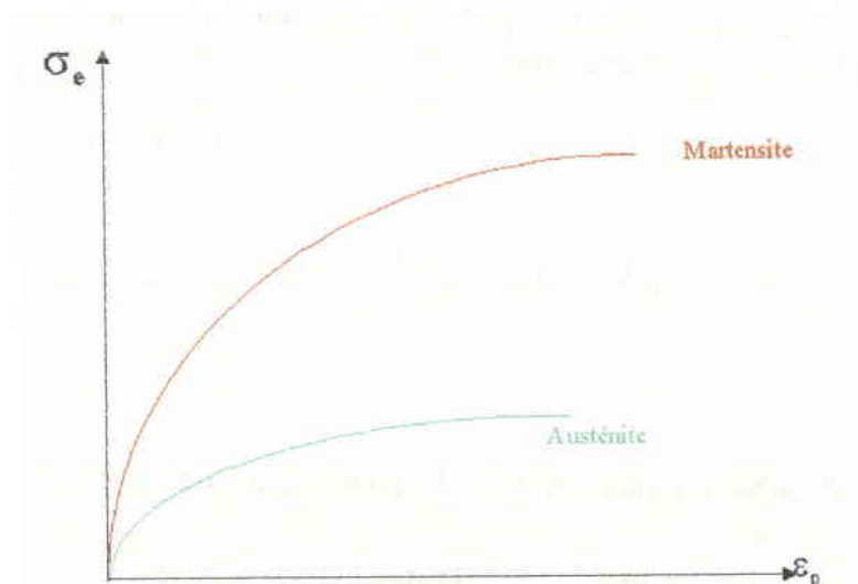
Figure VI.1 écouissage dans la phase austénitique et dans la phase martensitique
