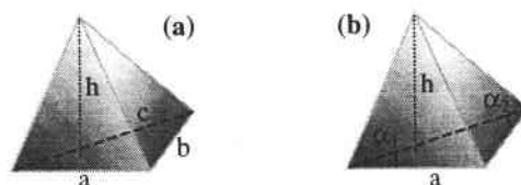
Figure 3-8. Deux manières différentes de représenter un tétraèdre : avec des dimensions (a) ou avec des angles (b)
