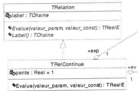
Figure 4-4. Classes du paquet estimation
