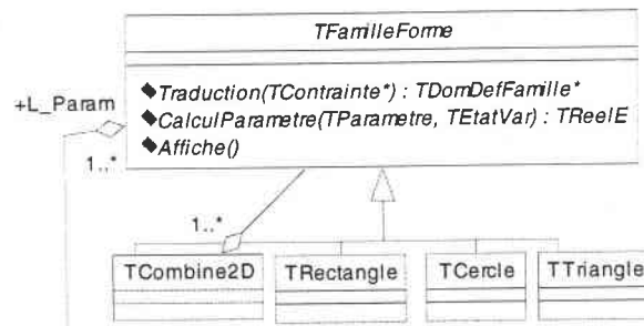
Figure 4-5. Classes du paquet bibliothèque de formes
