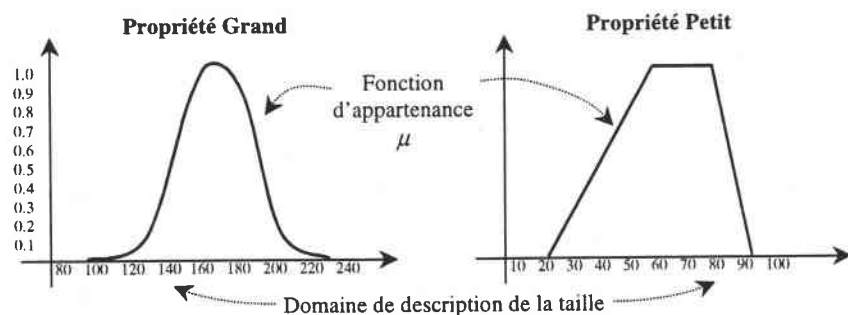
Figure 2-25. Principe d'association de la logique floue
