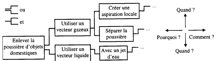
Figure 1-3. Diagramme FAST d'un aspirateur [Afav 89]
