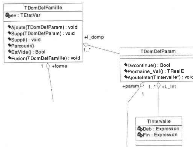
Figure 4-3. Classes du paquet espace des solutions
