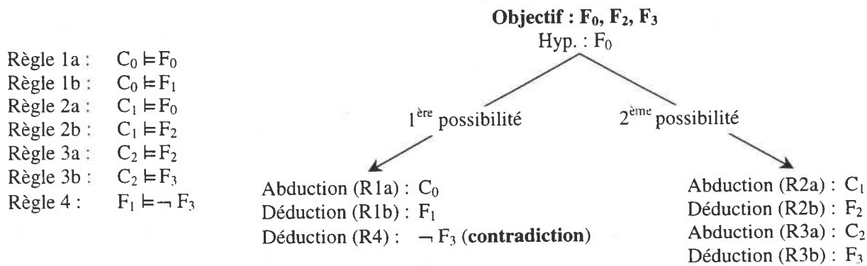
Figure 1-7. Application de déductions et d'abductions
