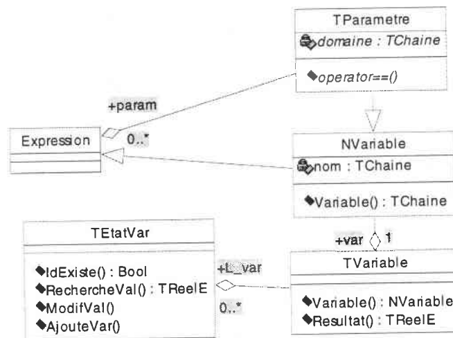
Figure 4-6. Classes du paquet expressions
