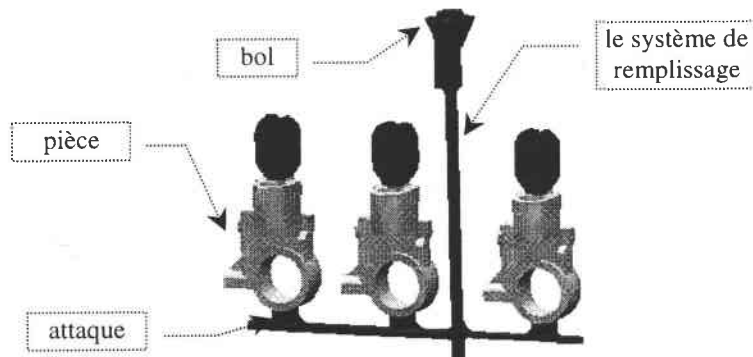
Figure 4-10. Composition d'un moule en fonderie 24
