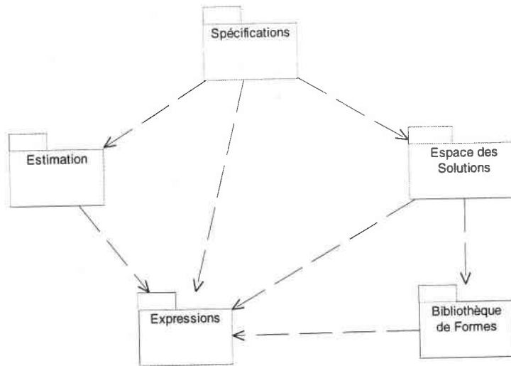
Figure 4-1. Diagramme des paquets
