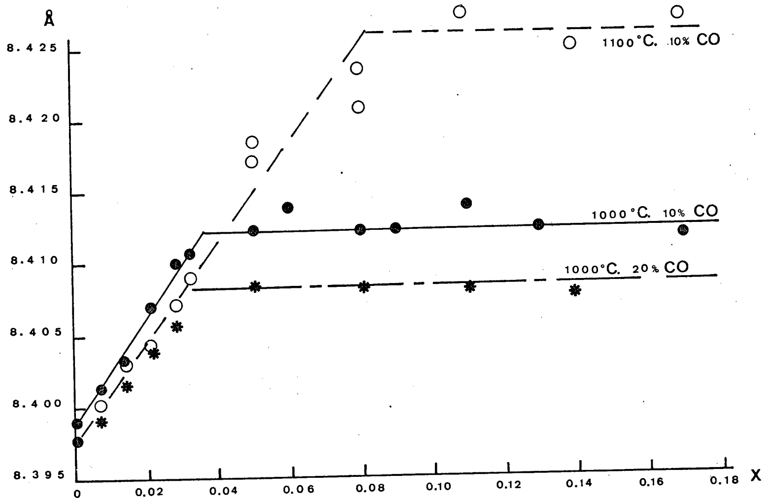
FIGURE II.2 EVOLUTION DU PARAMETRE CRISTALLIN DU SPINELLE (Fe_{1-x}Ca_x)O.Fe_2O_3 EN FONCTION DE x POUR DES TEMPERATURES DE 1000°C et 1100°C EN ATMOSPHERE CONTENANT 10 et 20 % DE CO ET 90 et 80 % de CO_2 . (d'après R. BLEIFUSS)
