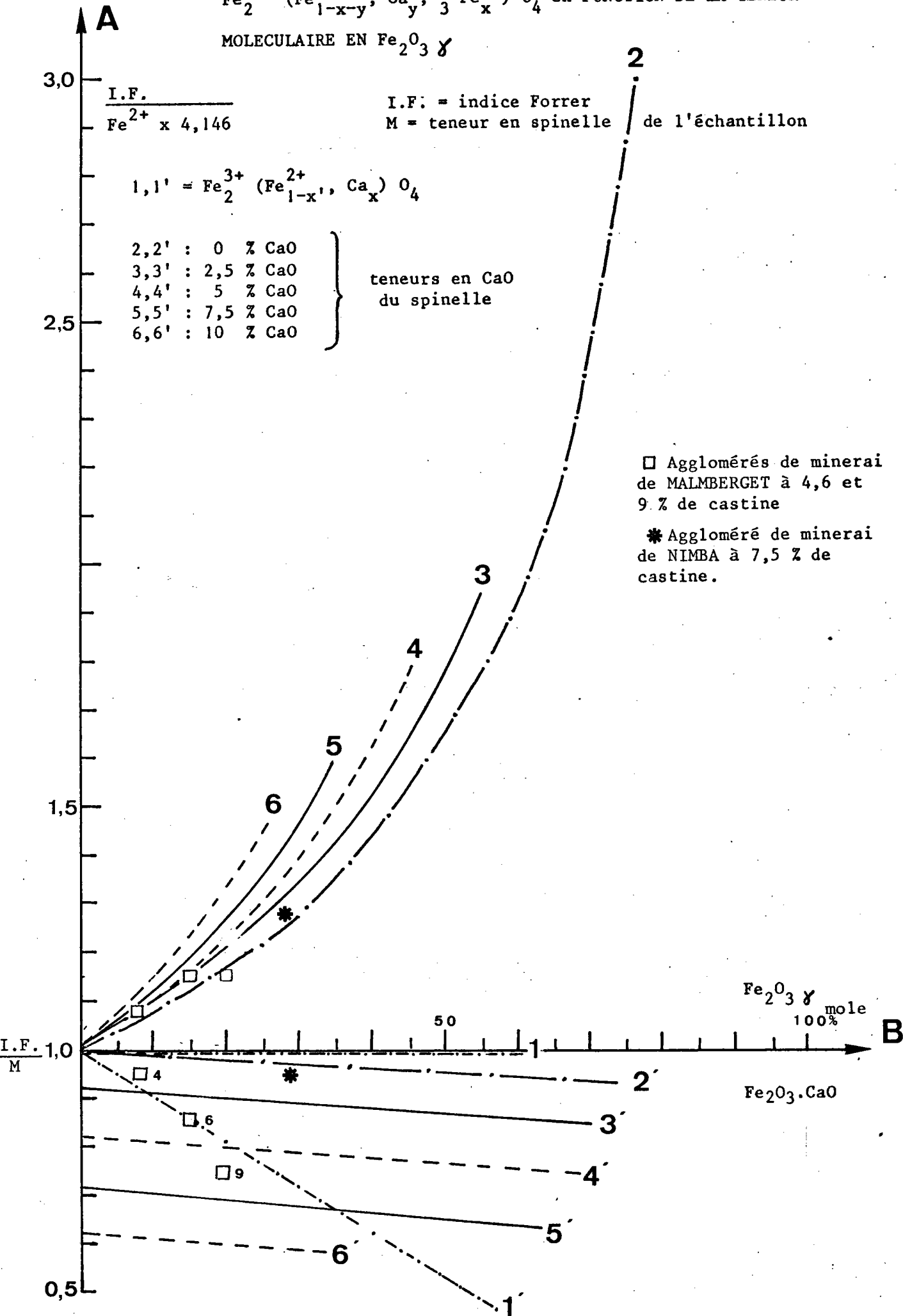
FIGURE V.15 - RAPPORT I.F./Fe 2+ x 4,146 et I.F./M DU SPINELLE
