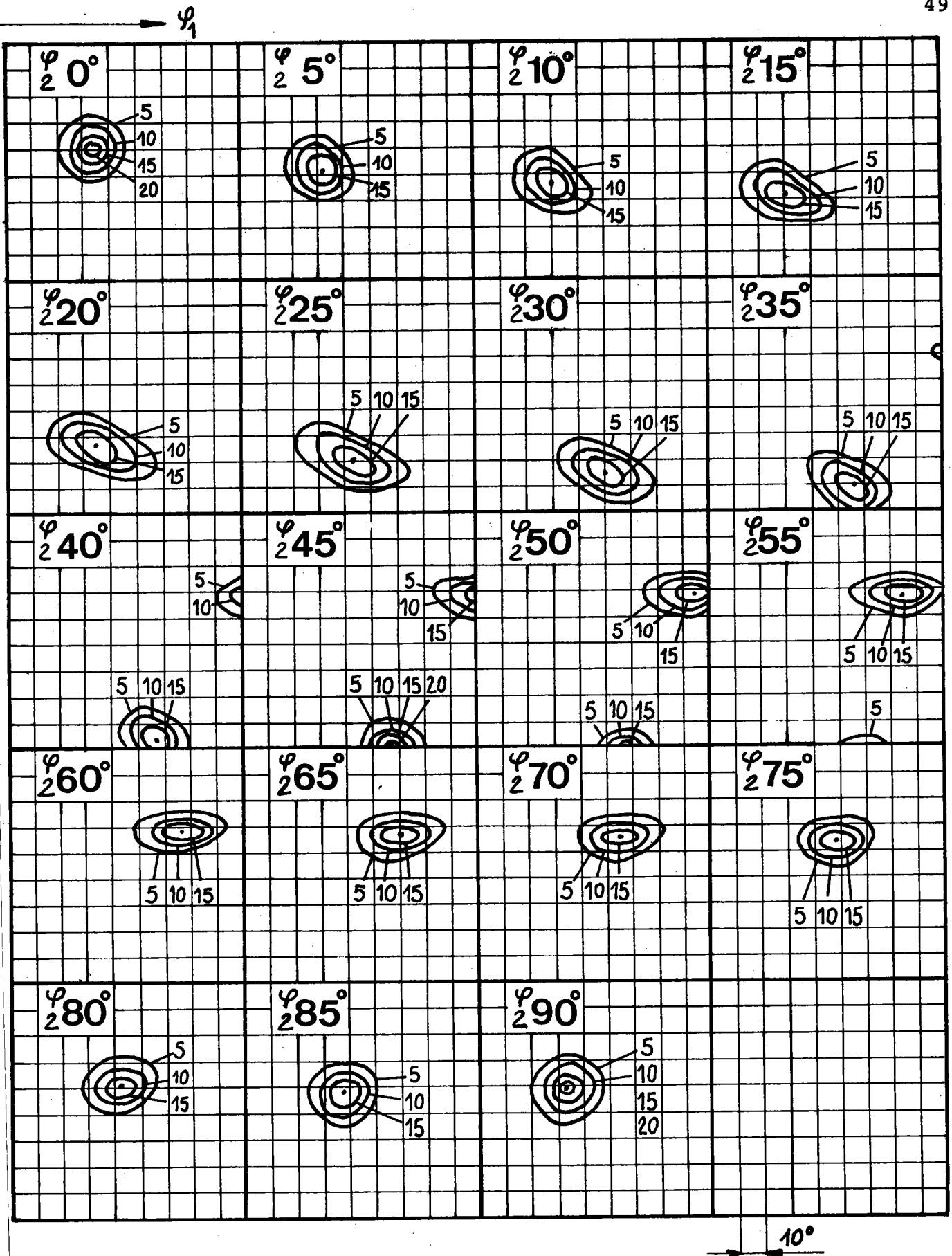
Fig. 25. Fonction de répartition des orientations de la texture de laminage du cuivre f(\psi_1, \phi \text{ et } \psi_2) d'après J. BUNGE ( \psi_1, \phi \text{ et } \psi_2 sont les angles d'Euler du repère formé par 3 axes \langle 001 \rangle dans les cristallites).
