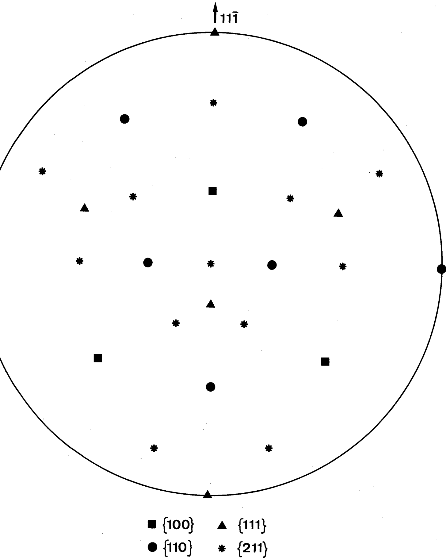
Fig. 20. Orientation (112) \angle \bar{111} \bar{1} .
