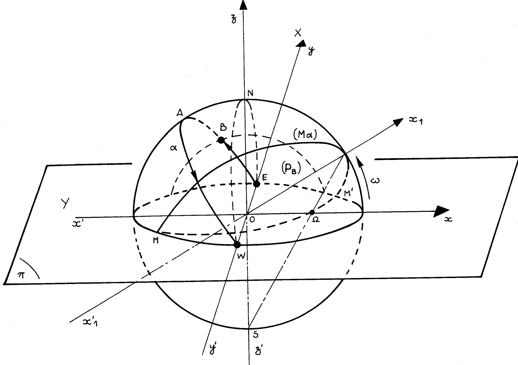
Fig.71. Projection stéréographique d'un méridien : le méridien (M_\alpha) se projette suivant l'arc \widehat{MOM'} .
