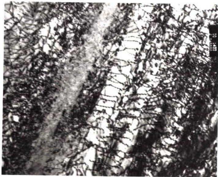
b - (x40 000) – Dislocations confinées dans leur plan de glissement
