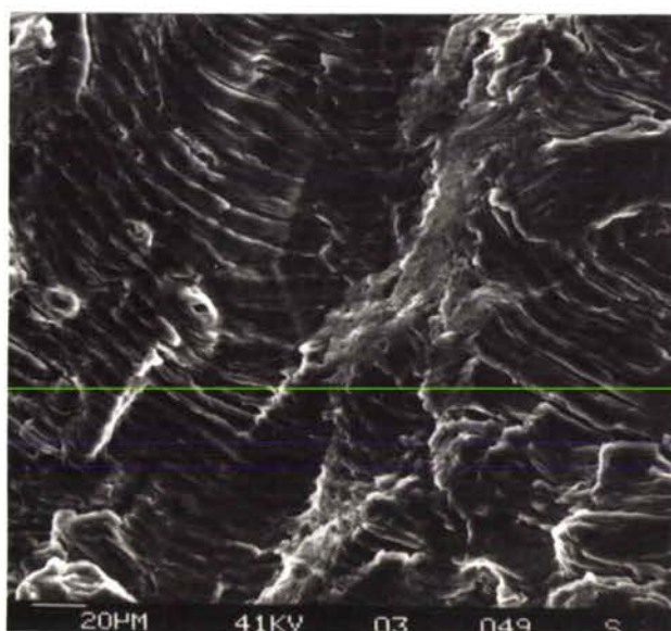
f - Stries de fatigue Éprouvette N2V10 : état vieilli
