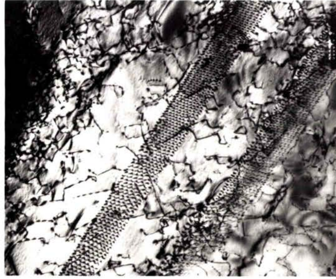
b - (x40 000) – Sous-joints de dislocations, t_m = 10\ 080 min
