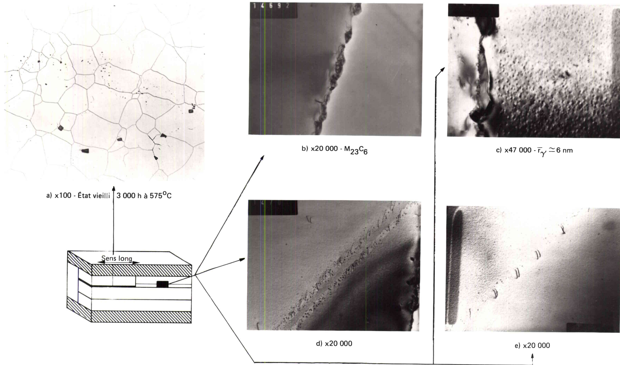
Figure III.7 – Structure du produit B108 grade 2 après vieillissement de 3000 h à 575°C.
