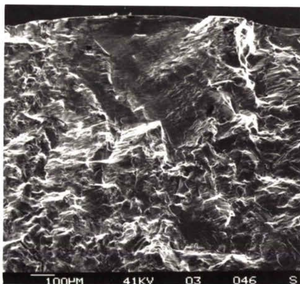
e - Site d'amorçage principal
