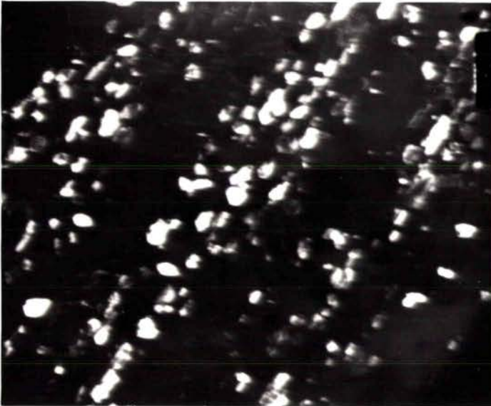
c - (x82 000) – Précipités de type M_{23}C_6 sur des bandes de déformation, t_m = 10\ 080 min
