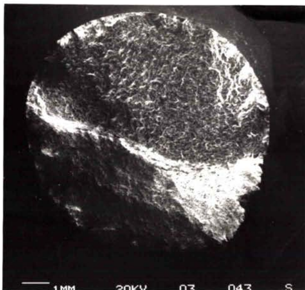
d - Aspect macroscopique
