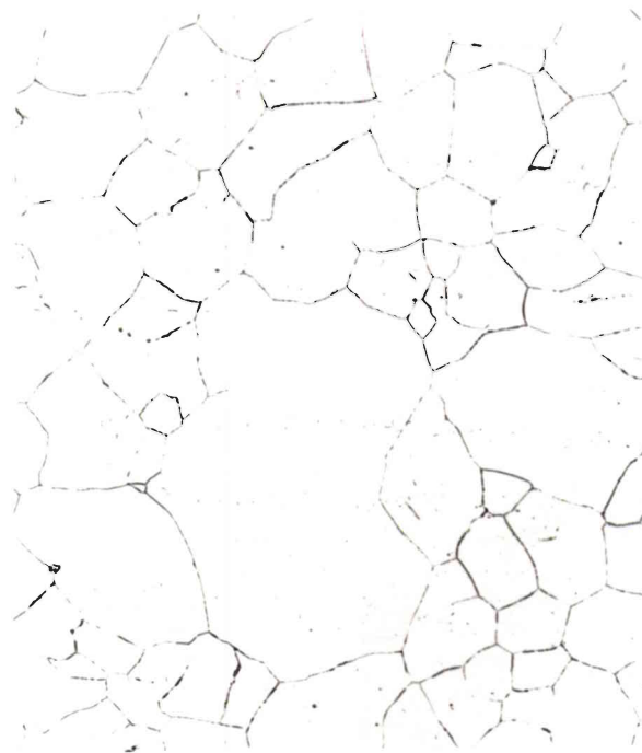
b) x200 - à cœur ; HV_{30} = 125 \pm 6
