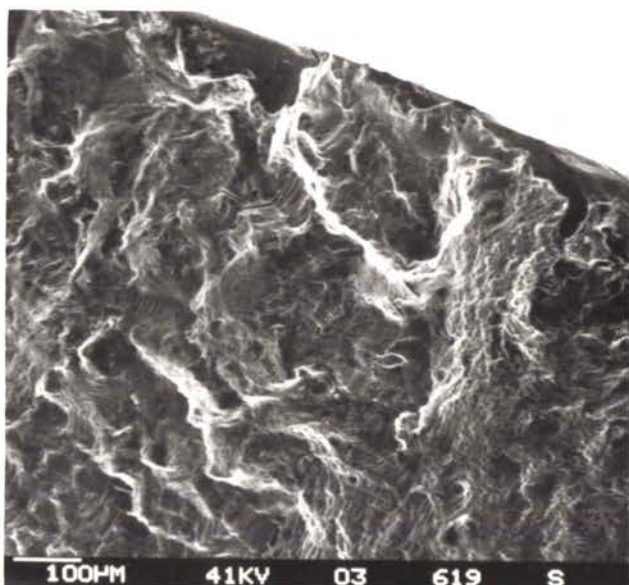
b - Site d'amorçage principal
