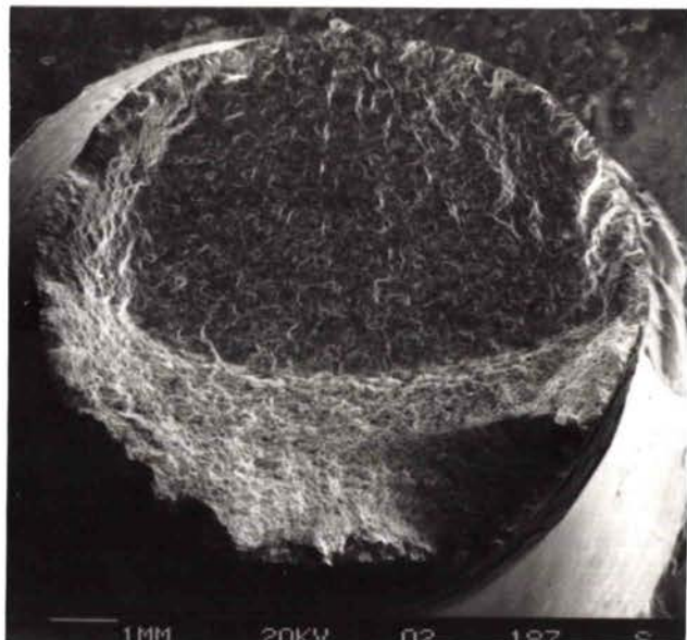
a - Aspect macroscopique
