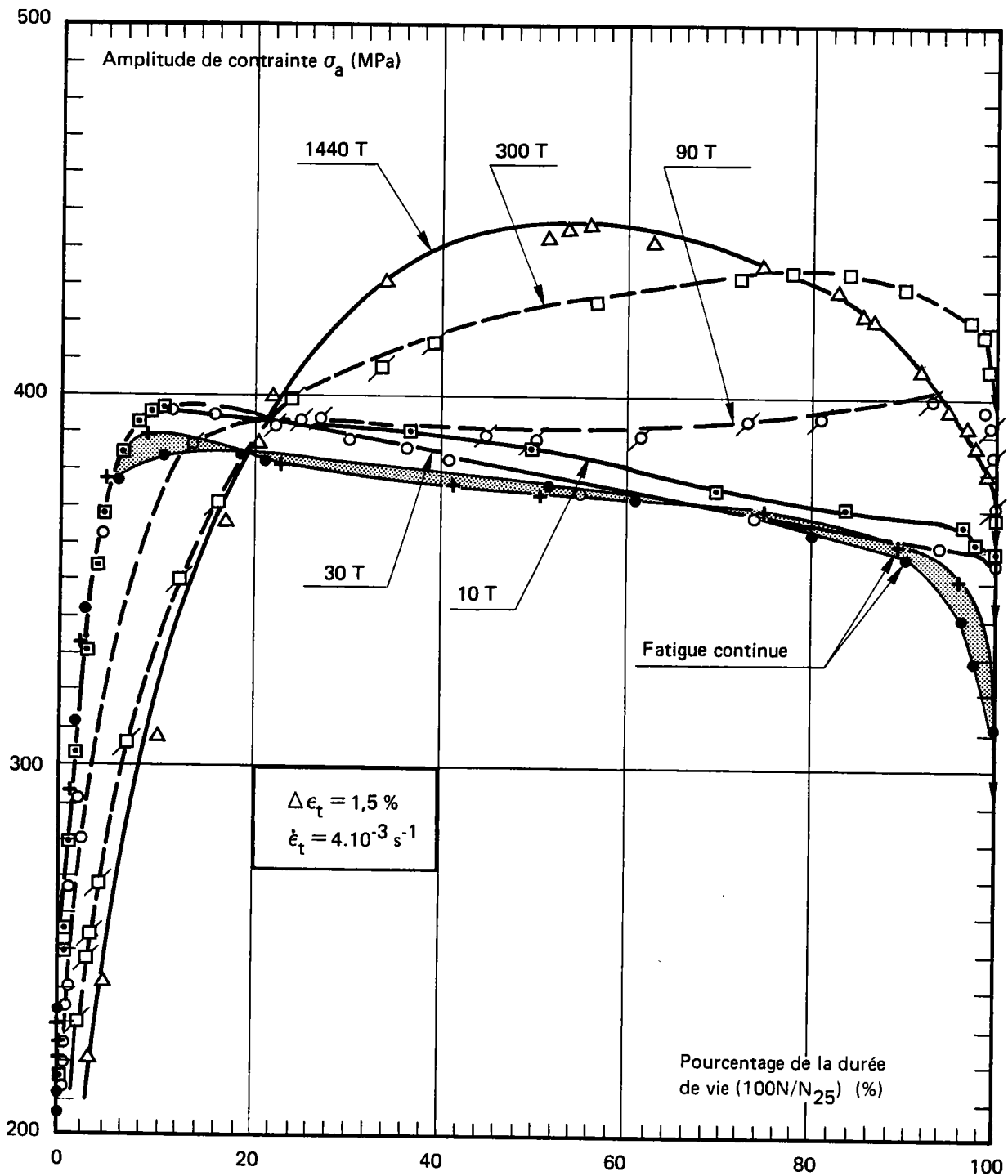
Figure V-13 — Évolution de l'amplitude de contrainte \sigma_a en fonction du pourcentage de la durée de vie (100N/N_{25}) . Alliage 800, grade 2 à l'état de réception. Fatigue-relaxation à 550°C avec maintien en traction.
