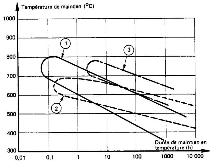
a — Essais comparatifs de corrosion intergranulaire sur Alliage 600, Alliage 800 et acier 316 à l'état hyperefflué
