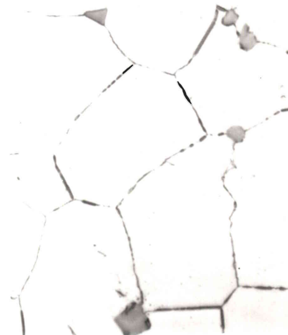
c) x1000 - à cœur
