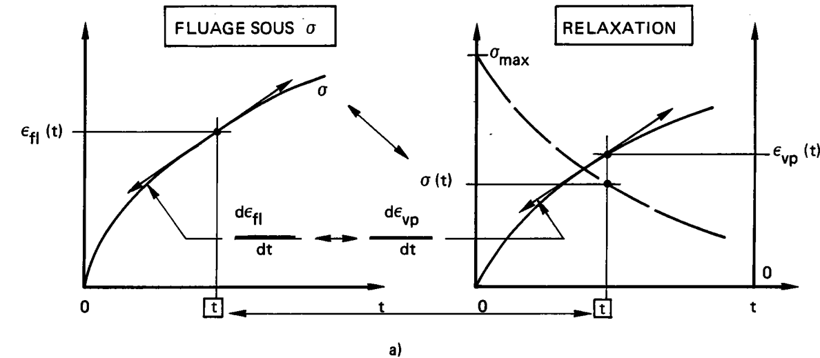
PASSAGE FLUAGE \Leftrightarrow RELAXATION DANS L'HYPOTHESE DU TIME-HARDENING
