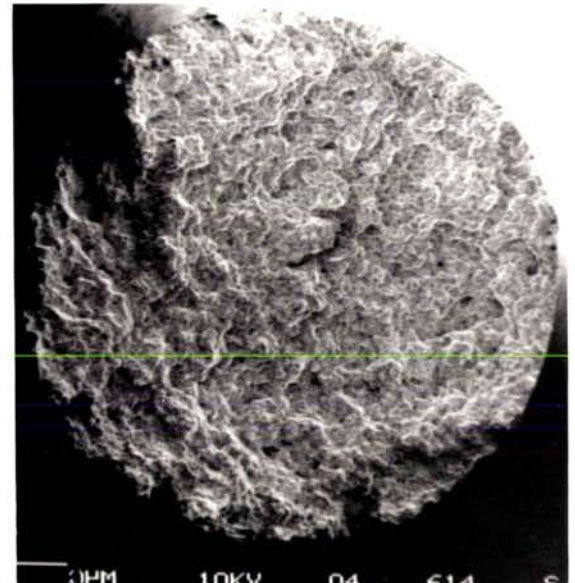
f - Fatigue-relaxation : éprouvette N2R58 ( t_{mt} = 1440 min)
