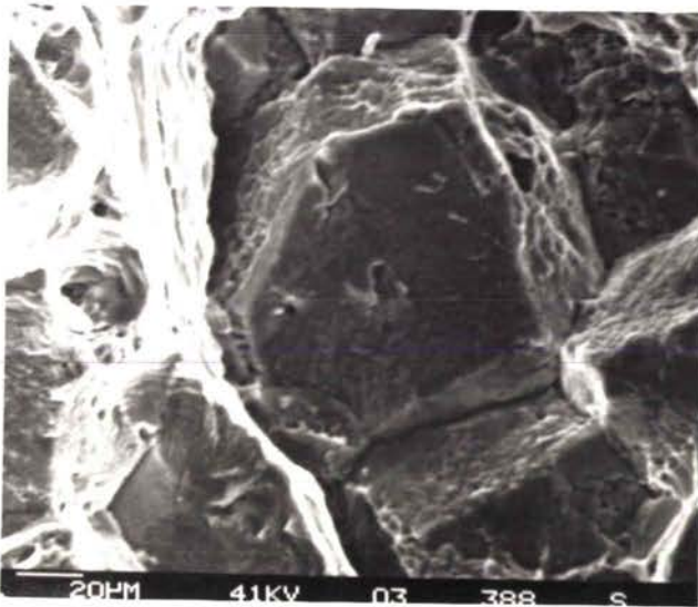
c - Décohésion intergranulaire
