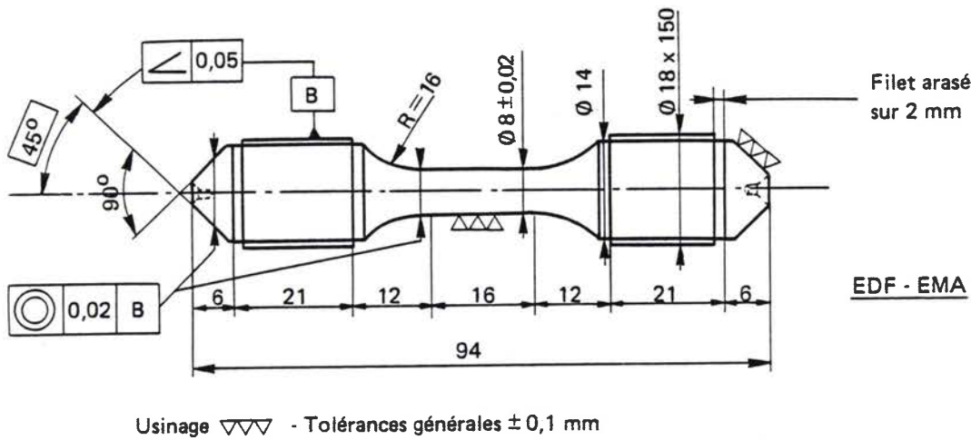
Figure V-2 – Éprouvette utilisée au Département EMA pour les essais de fatigue oligocyclique continue et de fatigue-relaxation.
