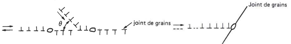
Figure V-34 – Mécanisme de base pour la germination de la décohésion intergranulaire en fluage, d'après B. Quantin (1981) [14].
