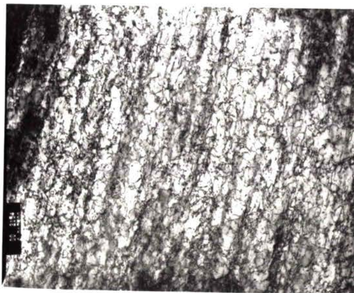
a - (x17 500) — Essai interrompu - Structure en bandes
