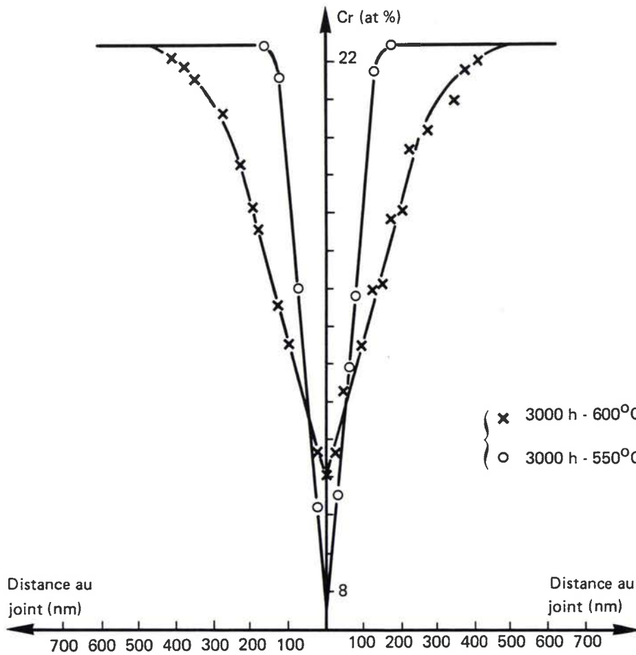
Figure III-12 — Profils de déchromisation après des maintiens de 3000 h à 550°C et 600°C.
