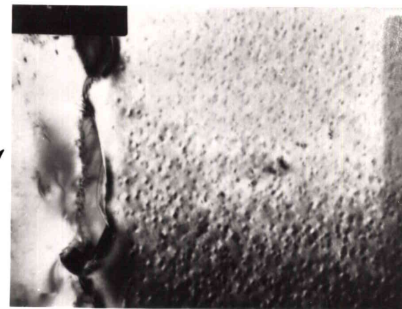
c) x47 000 - \bar{r}_{\gamma'} \simeq 6 \text{ nm}
