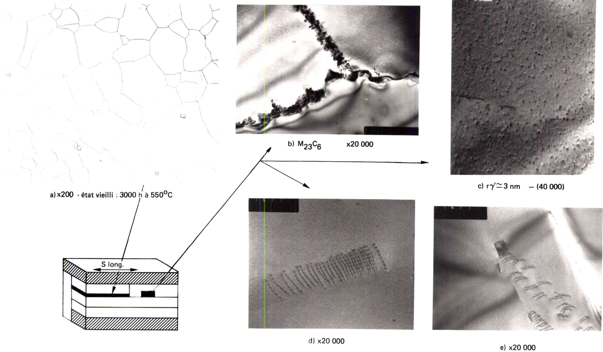
Figure III.6 — Structure du produit B108 grade 2 après vieillissement de 3000 h à 550°C.
