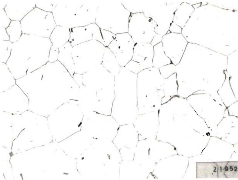
Figure III.1 - x200 – Micrographie à mi-épaisseur sur coupe transversale du plat B108-A en alliage 800 à l'état de grade 1 (état de réception). Attaque électrolytique à l'acide nitrique 20 %.
