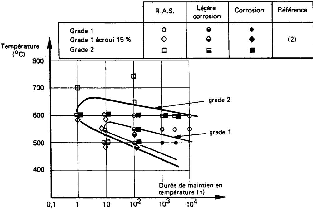
b — Résultats des essais de corrosion intercrystalline dans le réactif sulfo-cuprique après maintiens à différentes températures de la barre en l'état de grade 1 et 2
