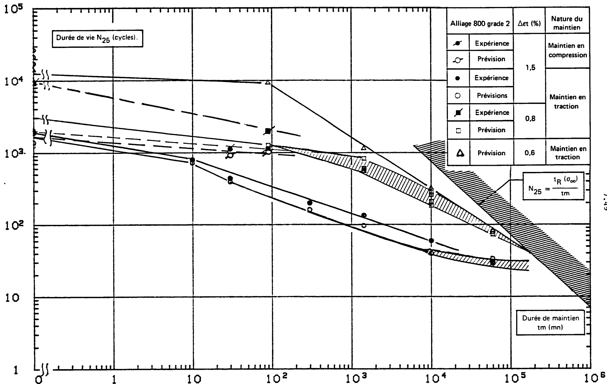
Figure VII - 12 — Résultats des prédictions de durée de vie à long terme à 550°C obtenues par le modèle ONERA en utilisant la loi de relaxation de Bui-Quoc modifiée avec l'hypothèse : n^{O_2} , sur la courbe de Woehler pour l'Alliage 800 grade 2 vieilli 3000 h à 550°C.
