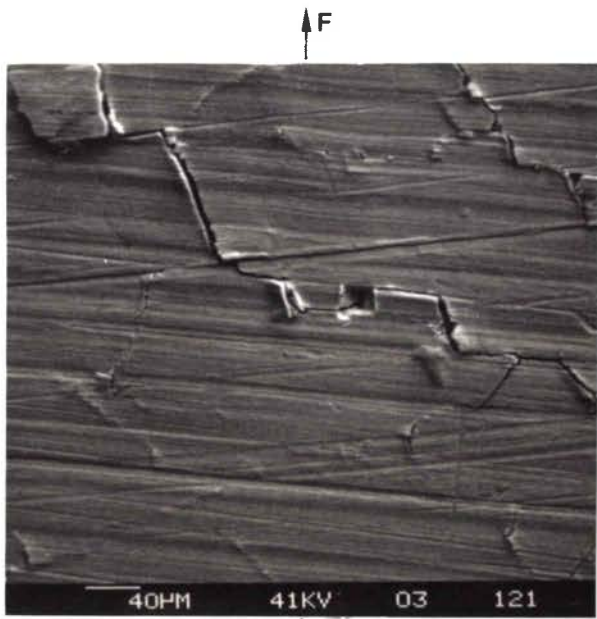
a - Éprouvette N2V10 - Fatigue continue
