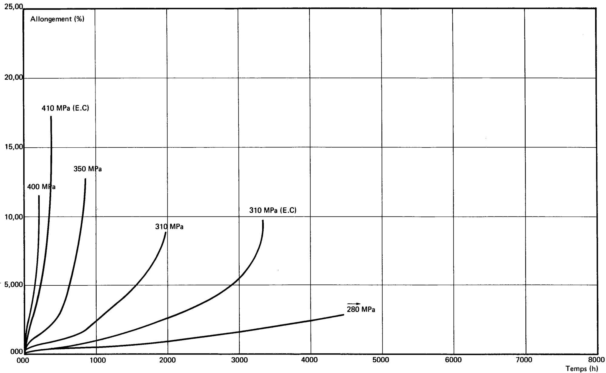
Figure IV-6 — Incoloy 800 - B108-A - Grade 2 vieilli 3000 h à 550°C — Courbes de fluage à 550°C sous différentes contraintes. (EC = fluage après écrouissage cyclique).
