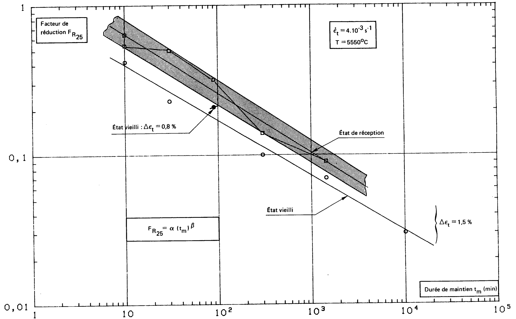
Figure V-23 – Évolution du facteur de réduction de durée de vie F_{R25} en fonction de la durée de maintien pour l'Alliage 800 grade 2 à 550^\circ\text{C} .
