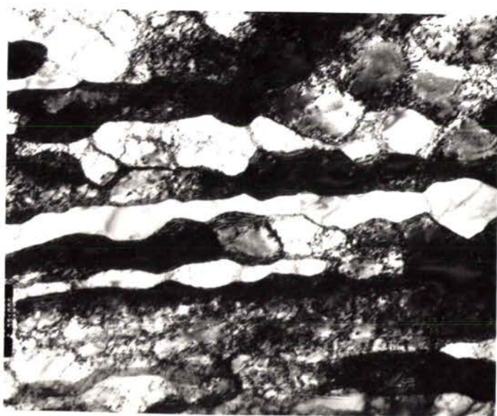
b - (x21 000) — Aspect général
