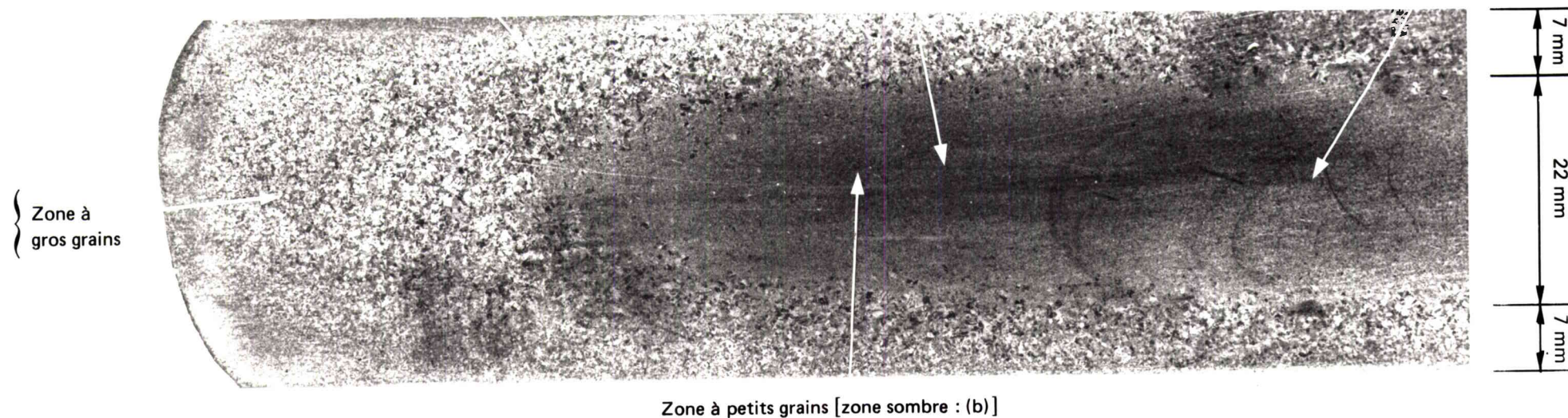
Figure III.2 – Structure micrographique du plat B108-A en état de grade 2 (état de réception) : étudiée sur coupe transversale après attaque électrolytique à l'acide nitrique à 20 % à 2 Volts.
