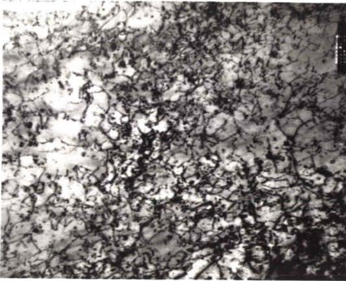
a - (x51 000) — Sous-structure de dislocations semi-homogène, t_m = 30 min
