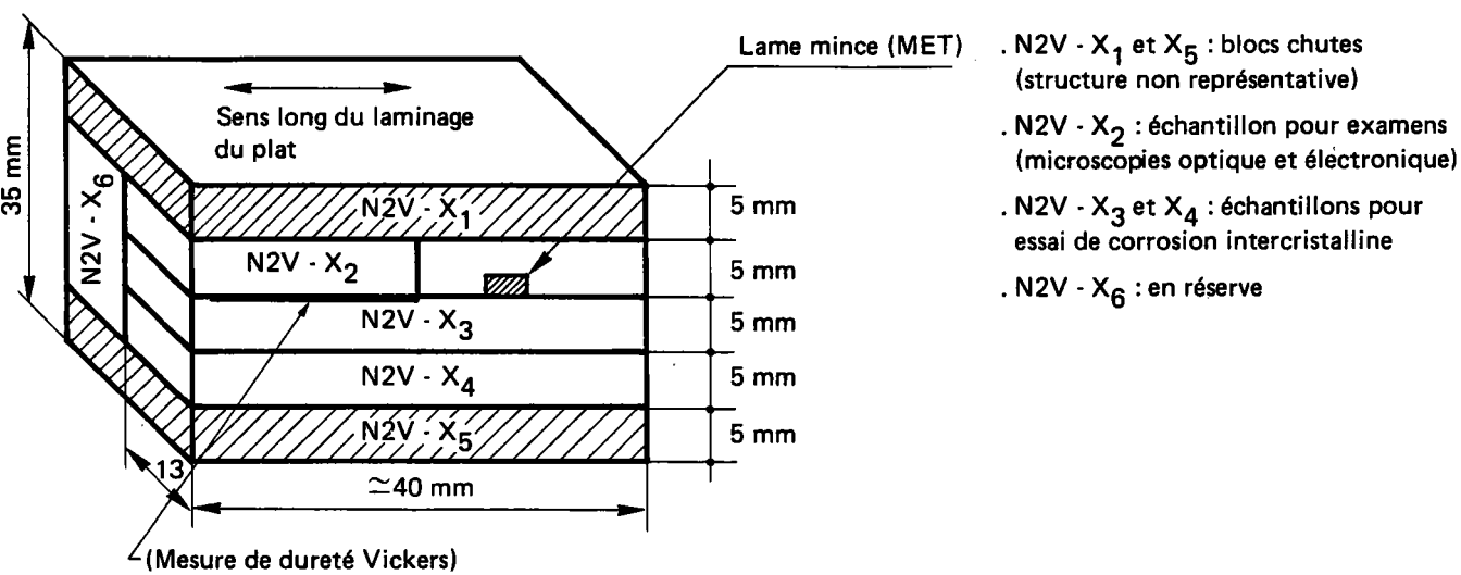
Figure III-4 – Plan de découpage des blocs après vieillissement.
