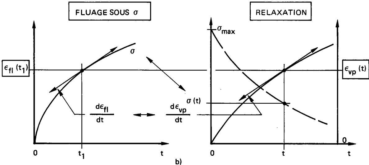
PASSAGE FLUAGE \Leftrightarrow RELAXATION DANS L'HYPOTHESE DU STRAIN-HARDENING
