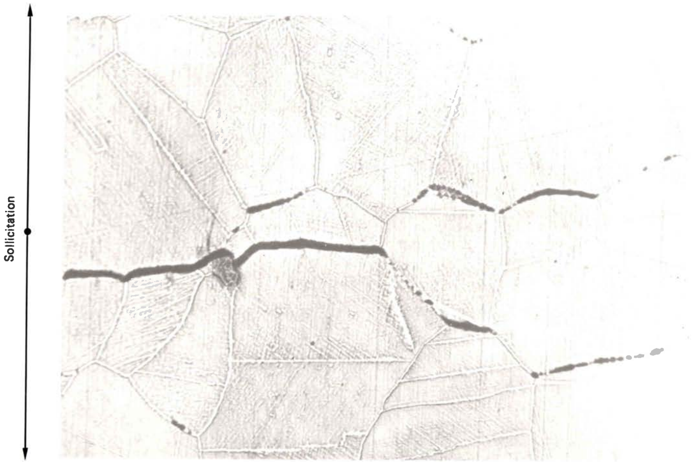
Figure V-33 — Aspects de la formation des décohésions intergranulaires sur coupe métallographique longitudinale. État vieilli, fatigue-relaxation, \Delta \epsilon_t = 1,5 \% - \theta = 550^\circ\text{C} - t_m = 10\,080 min en traction, éprouvette N2V30. Polissage électrolytique au réactif BEPER sous 40 V puis attaque électrolytique au Nital sous 2 V.
