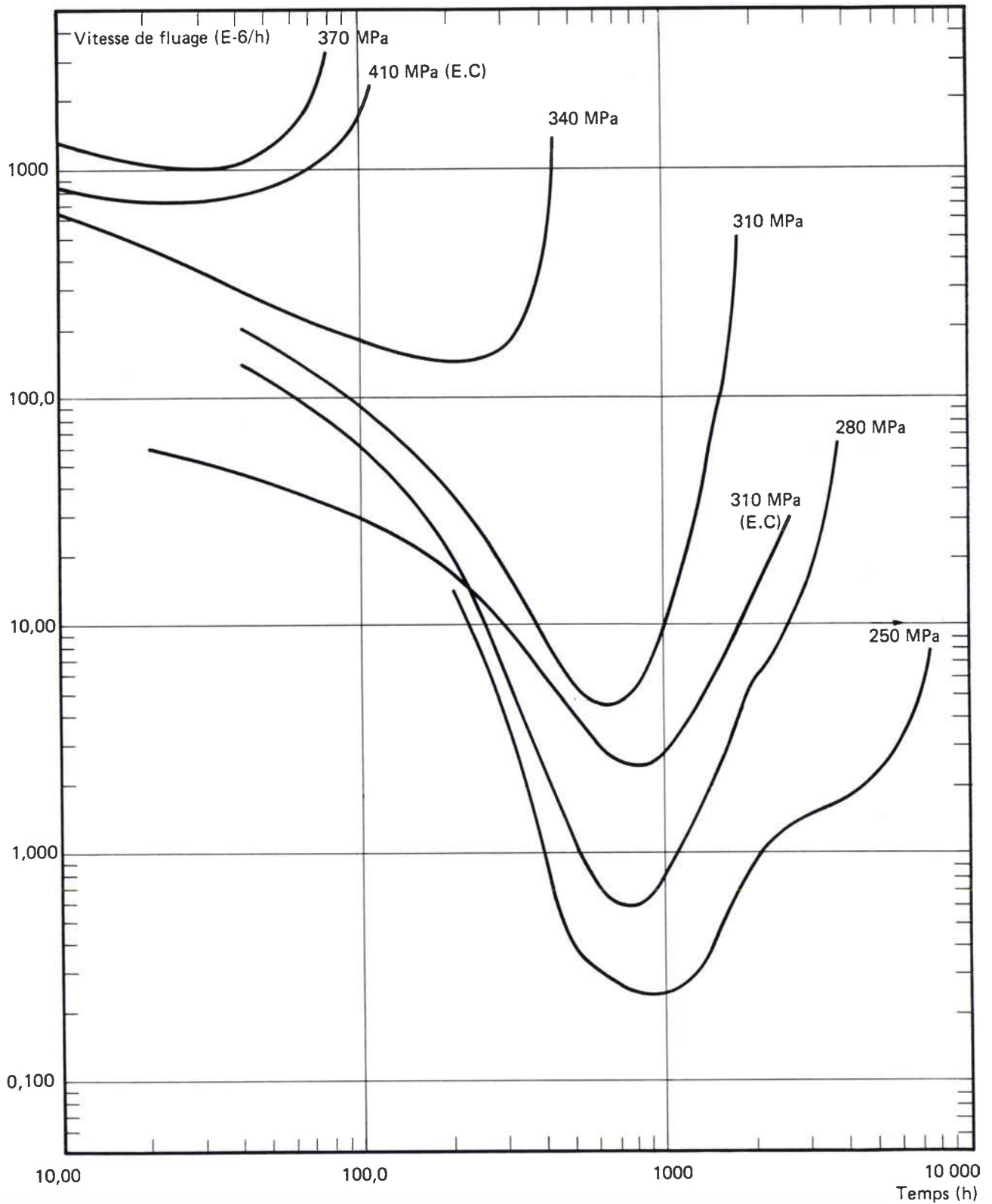
Figure IV-7 — Incoloy 800 - B 108-A - Grade 2 à l'état de réception — Évolution des vitesses de fluage à 550°C sous différentes contraintes. (EC = fluage après écrouissage cyclique).
