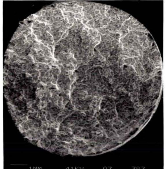
e - Fatigue-relaxation : éprouvette N2R29 ( t_{mt} = 300 min)
