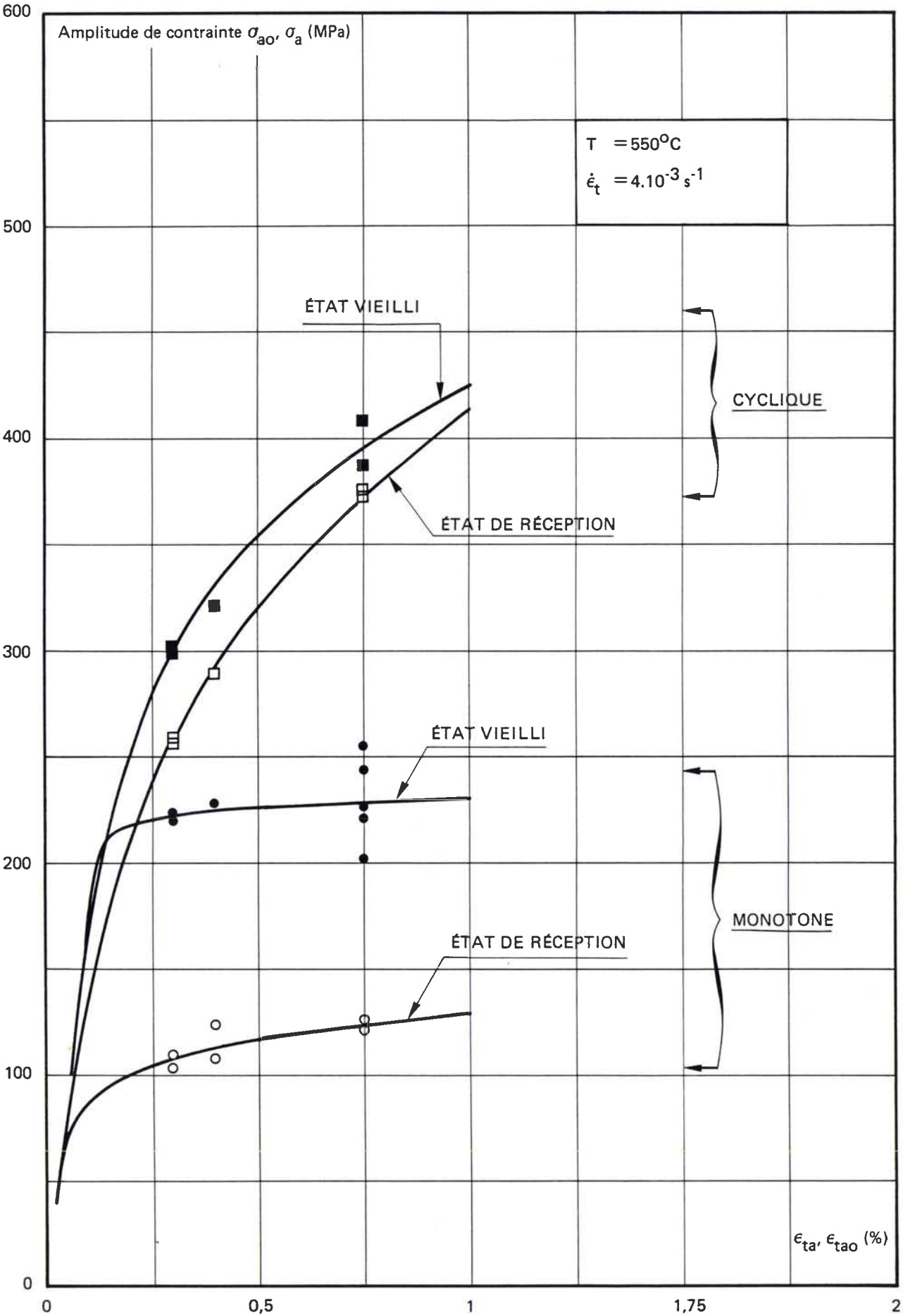
Figure V-7 – Comparaison des courbes de consolidation monotone et cyclique à 550°C de l'Alliage 800 grade 2 à l'état de réception et vieilli 3000 h à 550°C.
