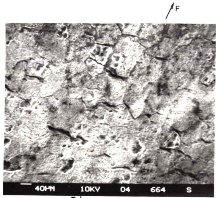
c - Éprouvette N2V30 - Fatigue-relaxation, t_m = 10\,080 min
