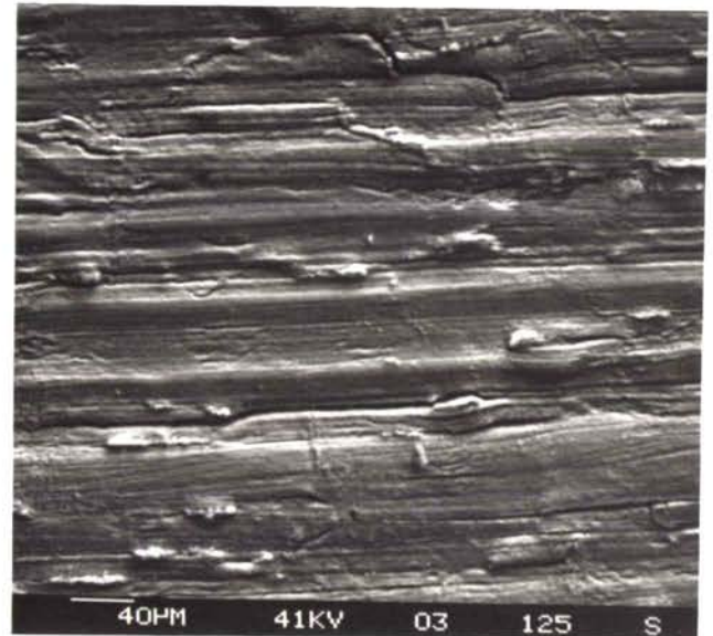
d - Loin de la rupture principale
