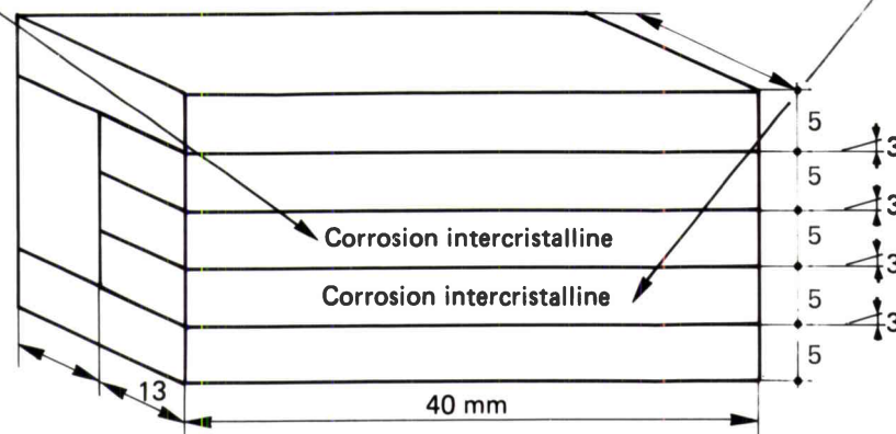
Figure III-10 — Prélèvement et aspect après pliage à 90° des éprouvettes d'essai de corrosion inter cristalline (matériau vieilli 3000 h à 525°C).
