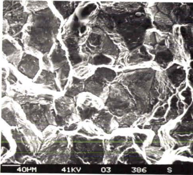
b - Endommagement intergranulaire au centre de l'éprouvette
