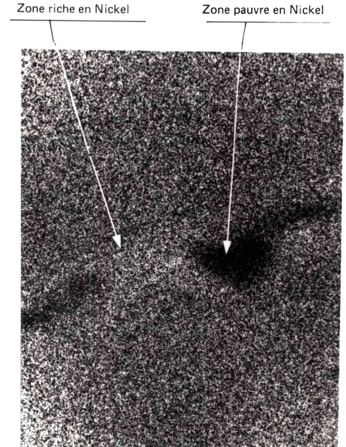
c) Image de répartition de la raie K_{\alpha} du Nickel
