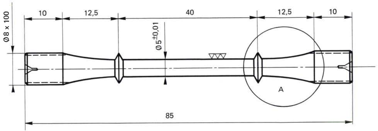
Détail A
