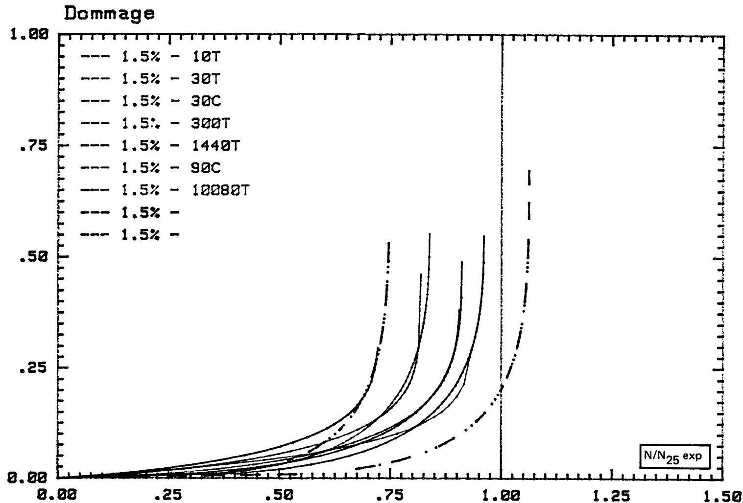
Figure VII - 10 — Évolution du dommage calculé par le modèle d'interaction fatigue-fluage de l'ONERA (D), en fonction du rapport ( N/N_{25 \text{ exp.}} ), pour des essais de fatigue continue et de fatigue-relaxation. Le calcul utilise la loi de relaxation de Bui-Quoc modifiée et les coefficients de fatigue du cas n°2 (cf. Tableau (VII - VII)).
