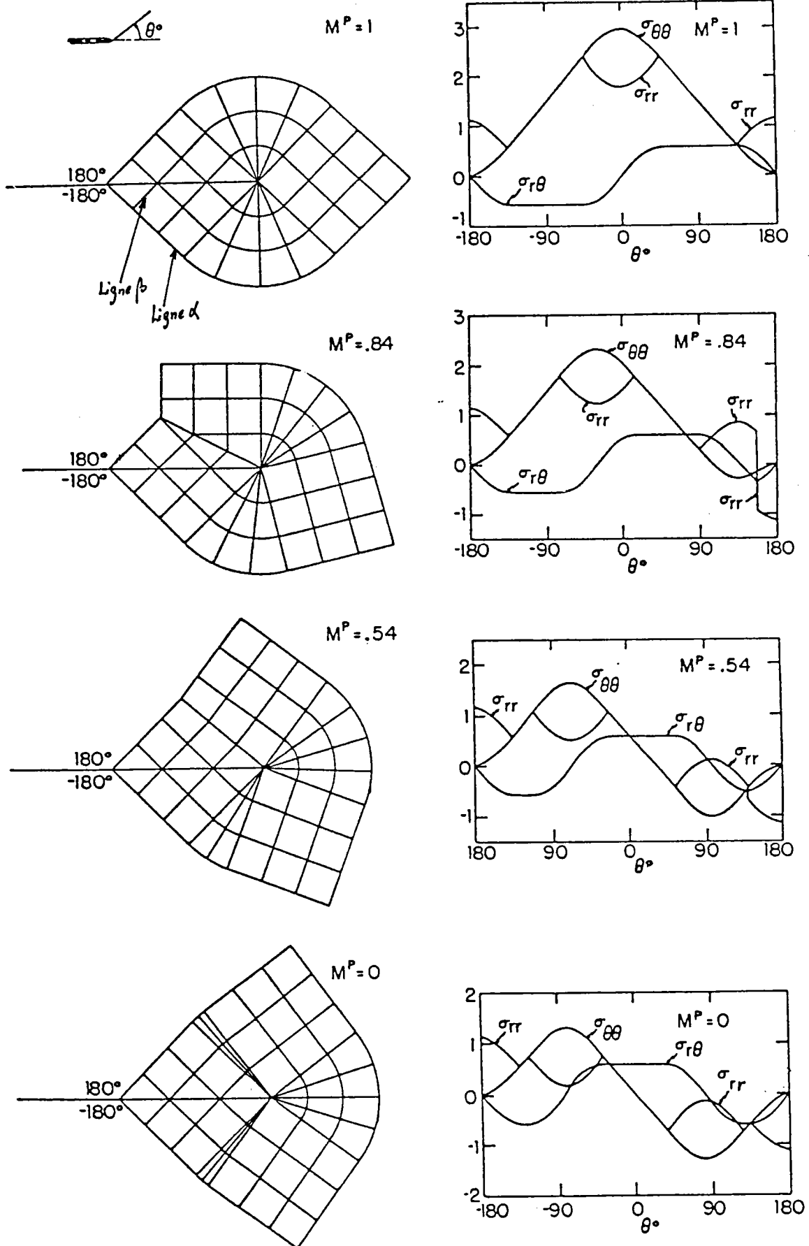
FIGURE (16) : Lignes de glissement et distribution des contraintes normalisés par rapport à \sigma_{\theta\theta} en pointe de fissure dans le cas de plasticité parfaite en déformation plane selon SHIH ((22))
