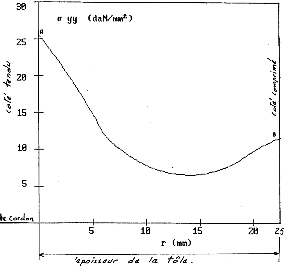
FIGURE (21) : Distribution des contraintes locales au pied de cordon à travers l'épaisseur.
