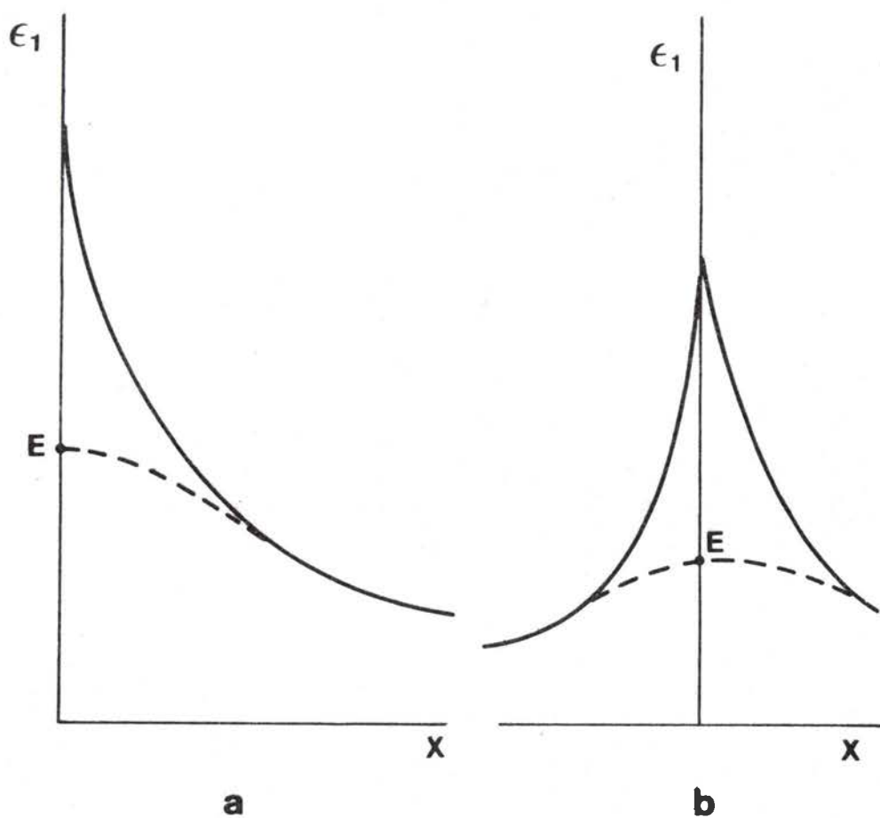
fig.A1/5 Méthode Bragard [6,7] d'extrapolation de la répartition des déformations à rupture.
