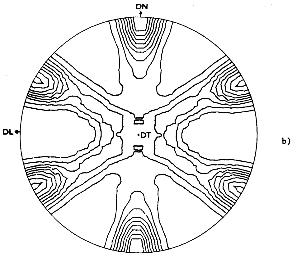
Fig. 40 : Figures de pôles d'axes OL et OT déduites de la figure de pôles expérimentale (111) incomplète représentée figure 19.
