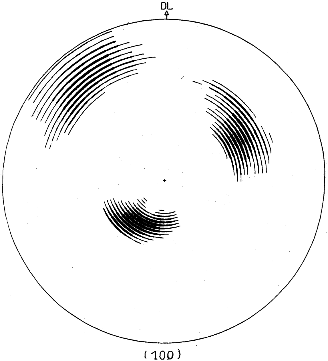
Fig. 17 : Figure de pôles représentant la distribution partielle A1. Cette composante correspond à environ 20 % du volume de l'échantillon.
