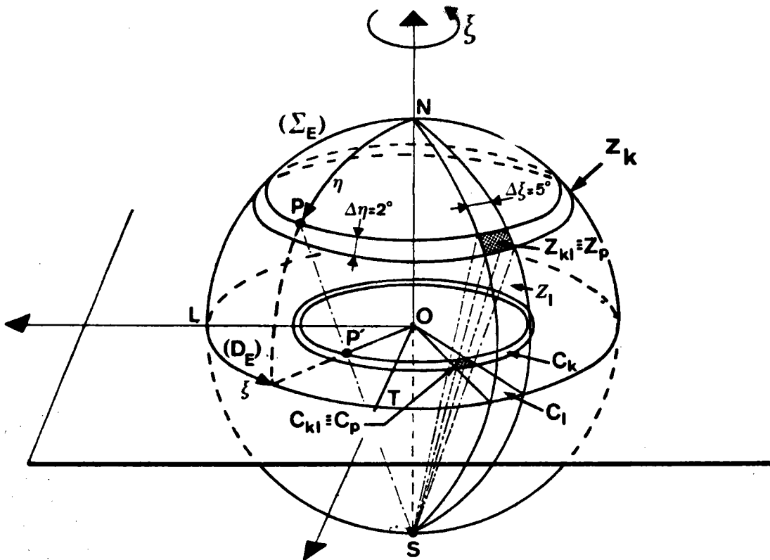
Fig. 7 : Partition de la demi-sphère des pôles (\Sigma_E) et de sa projection stéréographique (D_E) .
