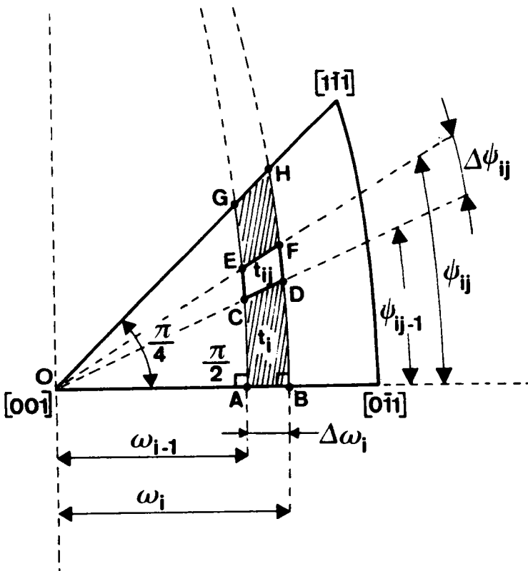
Fig. 34 : Une case t_{ij} ou t_\mu du triangle T_1 est définie comme l'intersection de deux fuseaux sphériques.
