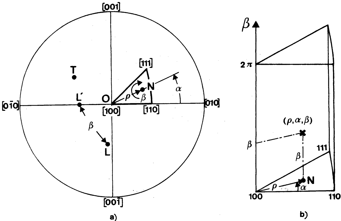
Fig. 2 : Définition des paramètres utilisés dans la méthode de R.O. WILLIAMS
