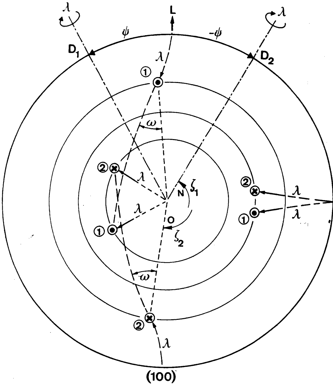
Fig. 6 : Différence de multiplicité des orientations et des fibres complètes.
