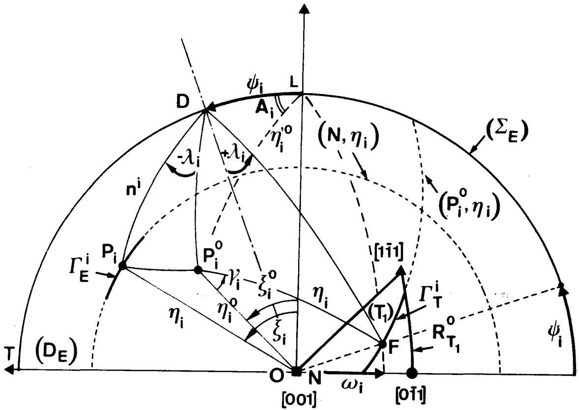
Fig. 8 : Relations géométriques entre les points de la figure de pôles inverse (T_1) et les pôles (hkl) représentés par les points P_i de (\Sigma_E) .
