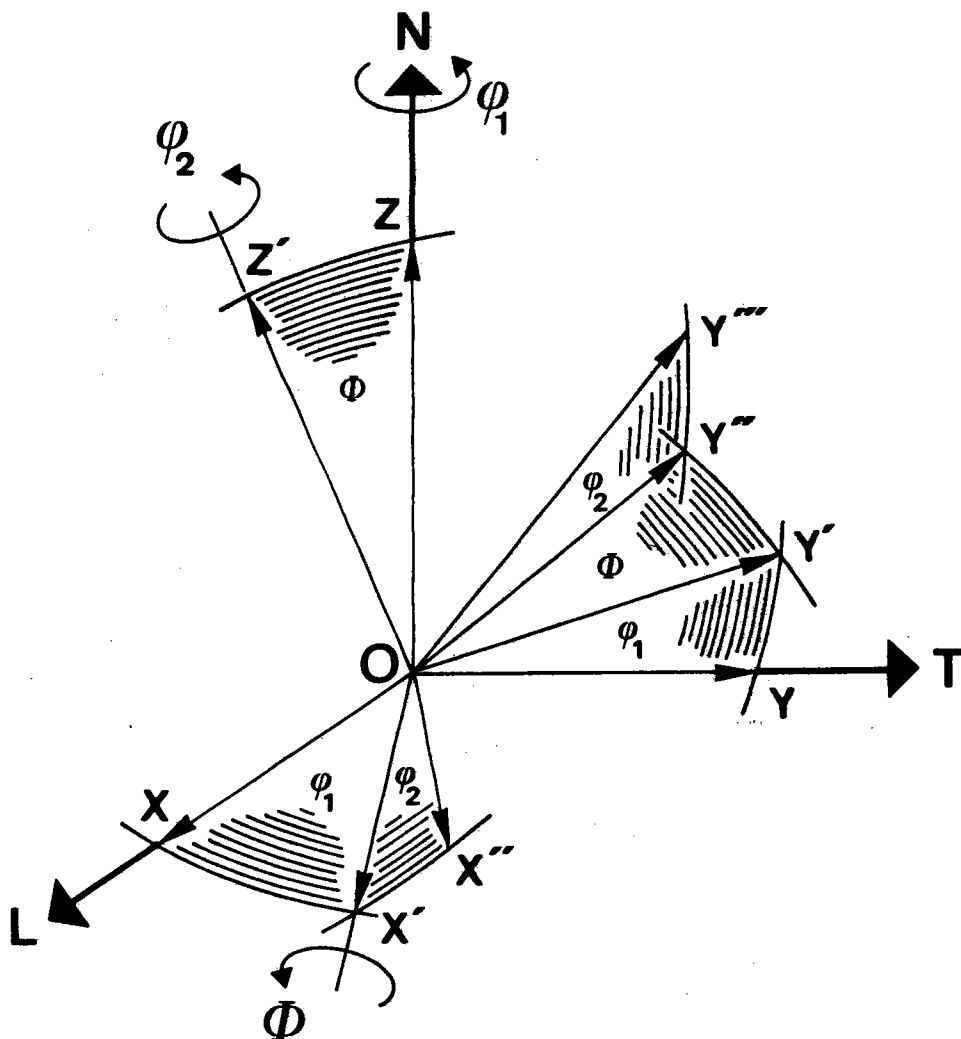
Fig. 1a : Définition des paramètres dans la méthode de H.J. BUNGE
