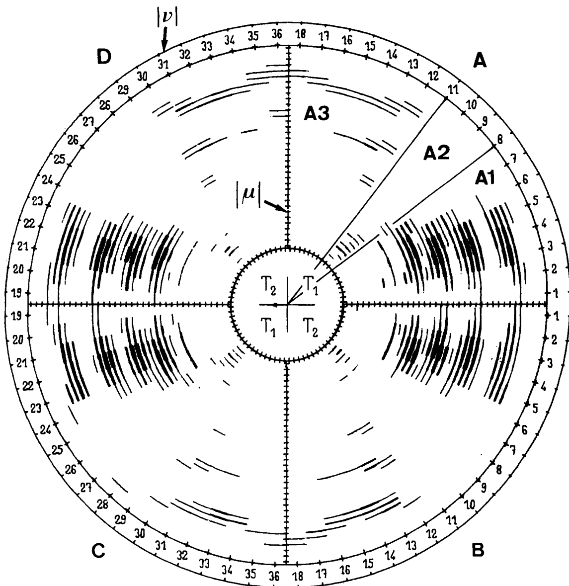
Fig. 16 : Représentation du vecteur Y reproduisant, lorsqu'elle existe, la symétrie orthorhombique de l'échantillon.
