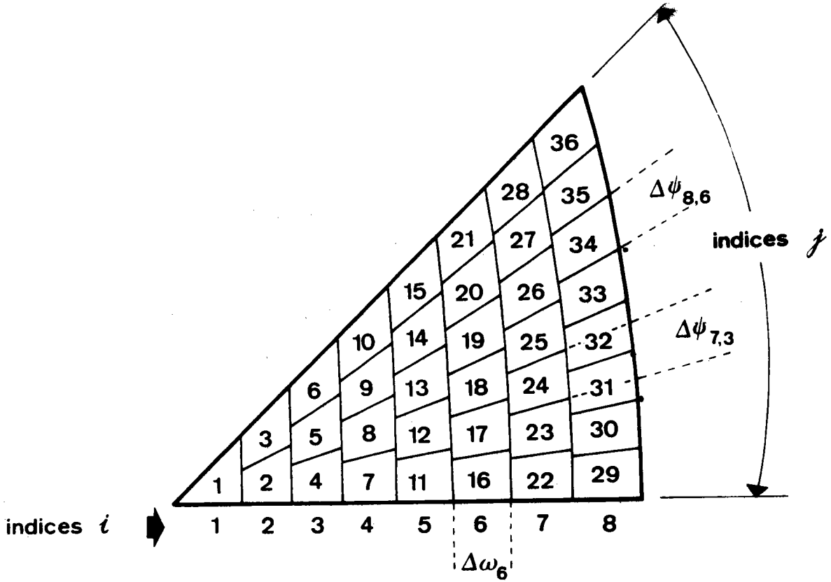
Fig. 4 : Partition du triangle sphérique T_1 en 36 cases t_\mu ( \mu=1, \dots, 36 ) d'aire égale. L'indice \mu est égal à i(i-1)/2 + j .
