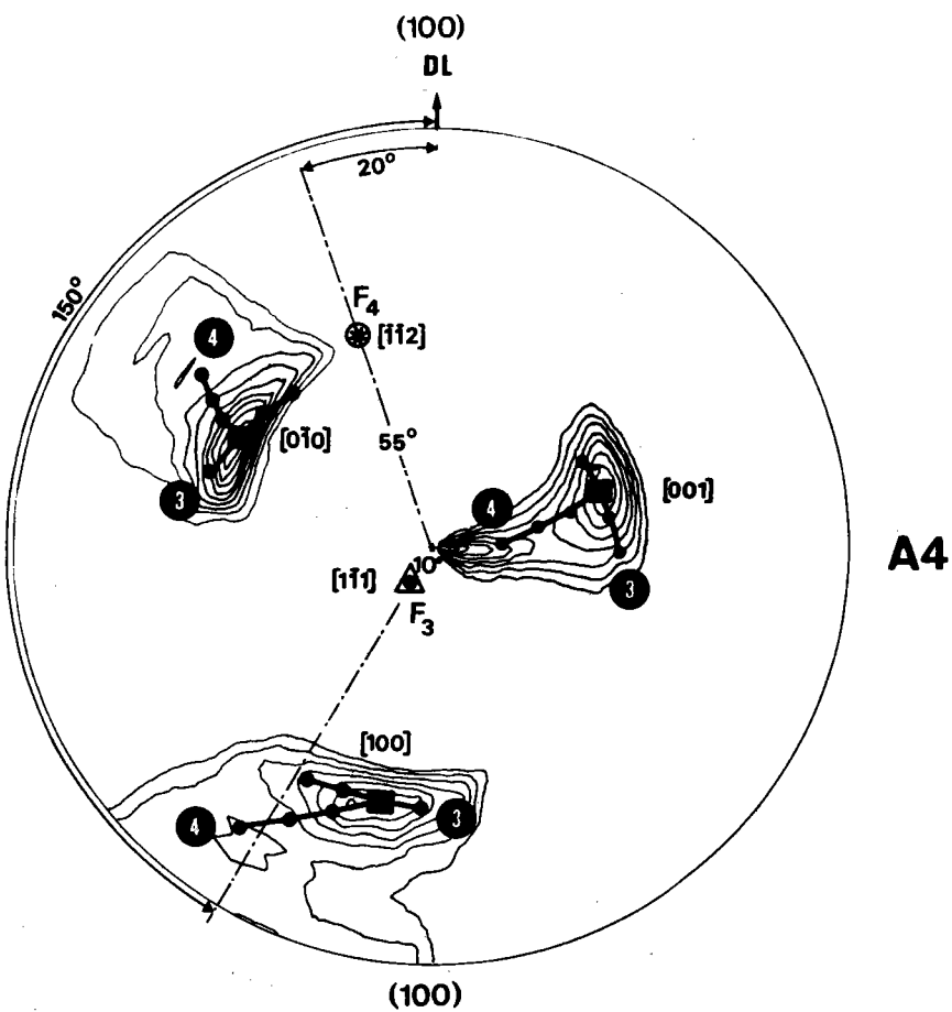
Fig. 30 : Analyse qualitative des composantes A3 et A4.
