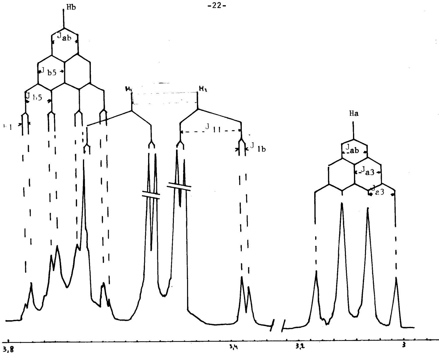
Agrandissement du spectre de 5(0,0) entre 2,8 et 3,8 ppm
