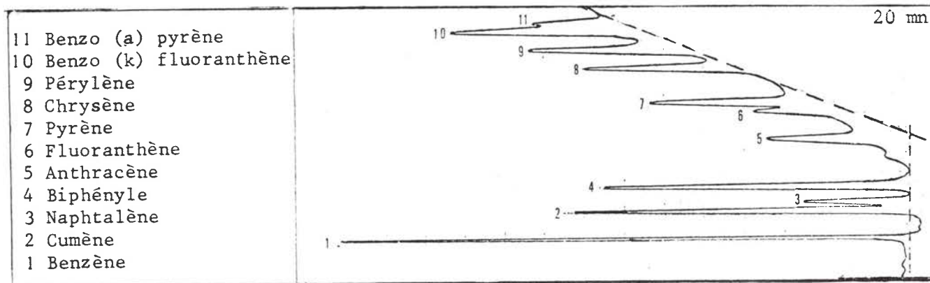
Figure 7 : chromatogramme d'un mélange synthétique de polyaromatiques Colonne DDS permaphase gradient d'éluion \text{CH}_3\text{OH}-\text{H}_2\text{O} : 50-50 à \text{CH}_3\text{OH}-\text{H}_2\text{O} : 95-5 à 2 % / mm. Débit 54 ml/h.
