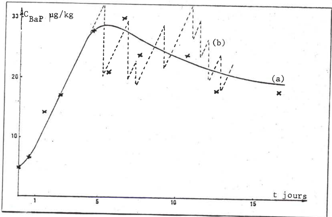
Figure 41: Enrichissement en benzo(a)pyrène au cours du temps; (a) allure générale — (b) allure théorique en fonction des ajouts ----
