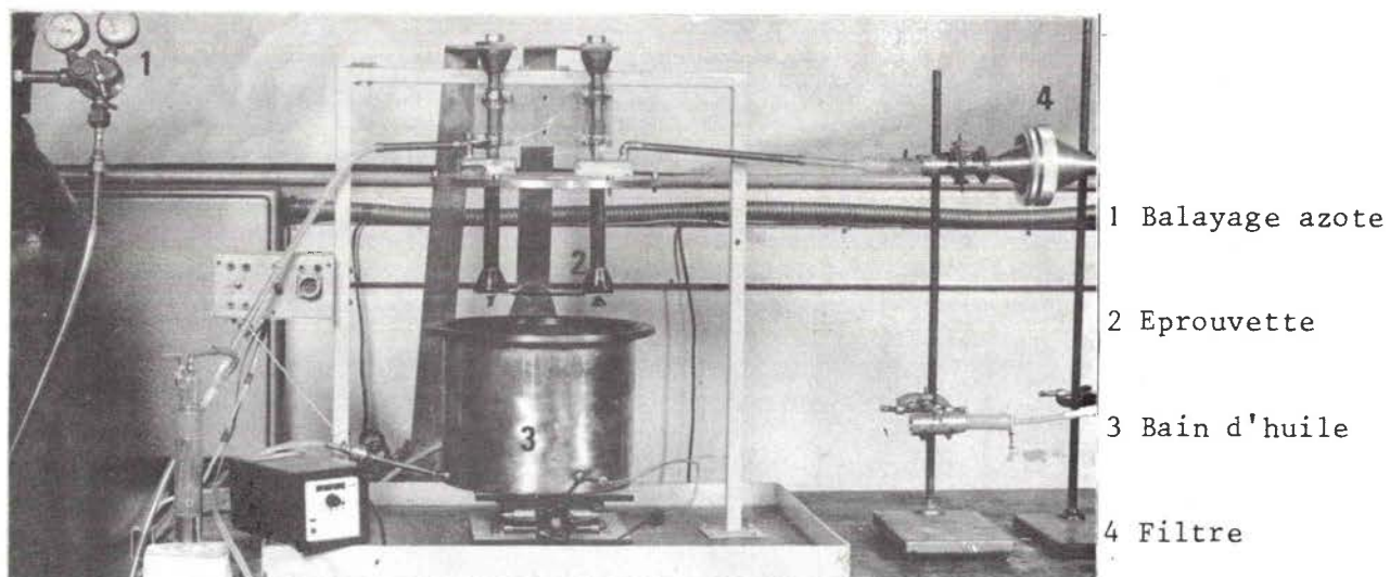
Montage expérimental
