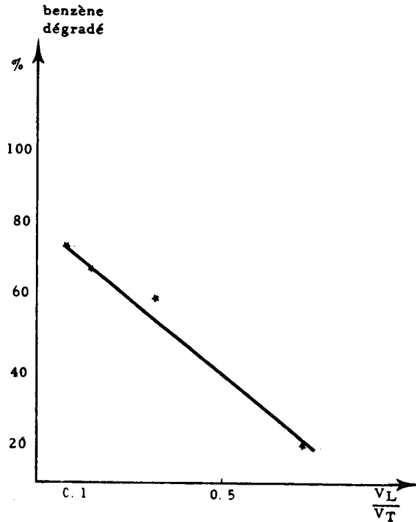
Figure n° 29 : Dégradation du benzène par la souche M influence de la quantité d'oxygène disponible V_L : volume du liquide V_T : volume total du flacon
