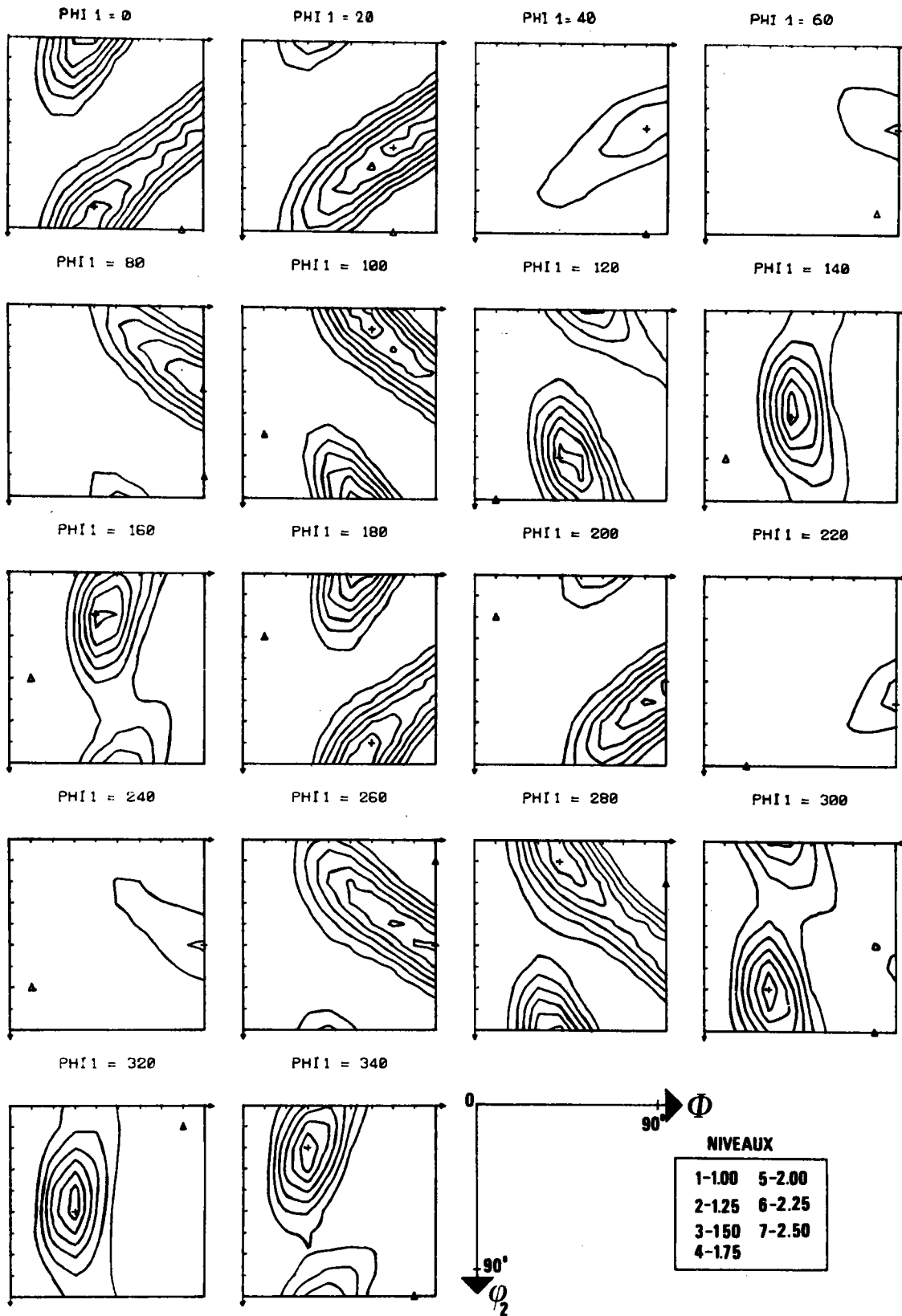
Fig. 3.9. : Section à \psi_1 = \text{cste} de la fonction de texture pour l'échantillon de magnétite.
