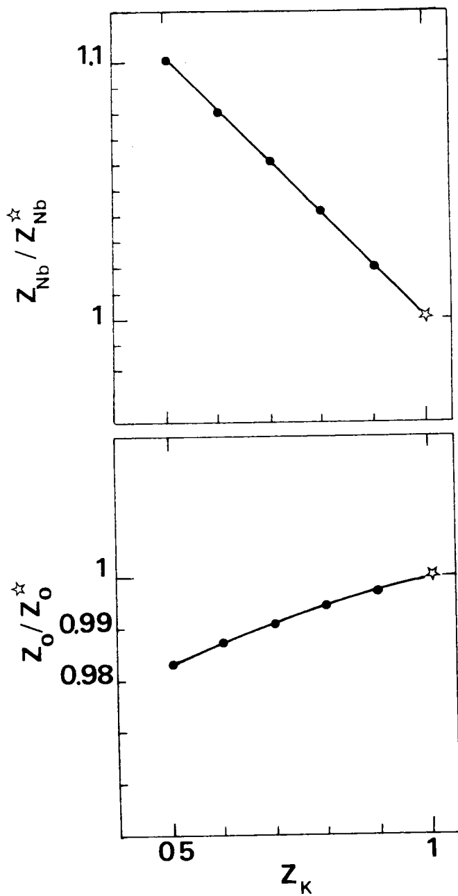
FIGURE 6.1 : Variation relative des charges effectives du niobium et de l'oxygène en fonction de la valeur Z_K de la charge effective du potassium. Z_O^* et Z_{Nb}^* se réfèrent aux valeurs prises lorsque Z_K = 1 .
