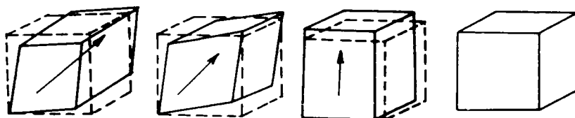
FIGURE 6.6 : Description des transitions successives de \text{KNbO}_3 : la séparation du mode FE T01 en composantes dures et molles, lors de chaque transition structurale, est connectée à une distorsion de la maille cristalline et à une réorientation de P_S .
