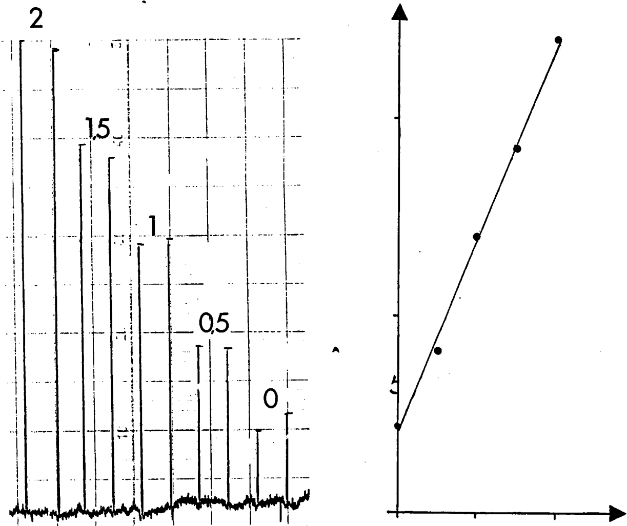
FIG. 40 : ENREGISTREMENT D'UNE GAMME D'ÉTALONNAGE MONTANTE ENTRE 0 ET 2 µg/L DANS DU MILIEU OLIGO L.C. (À GAUCHE). TRACÉ DE LA DROITE D'ÉTALONNAGE CORRESPONDANTE (À DROITE).
