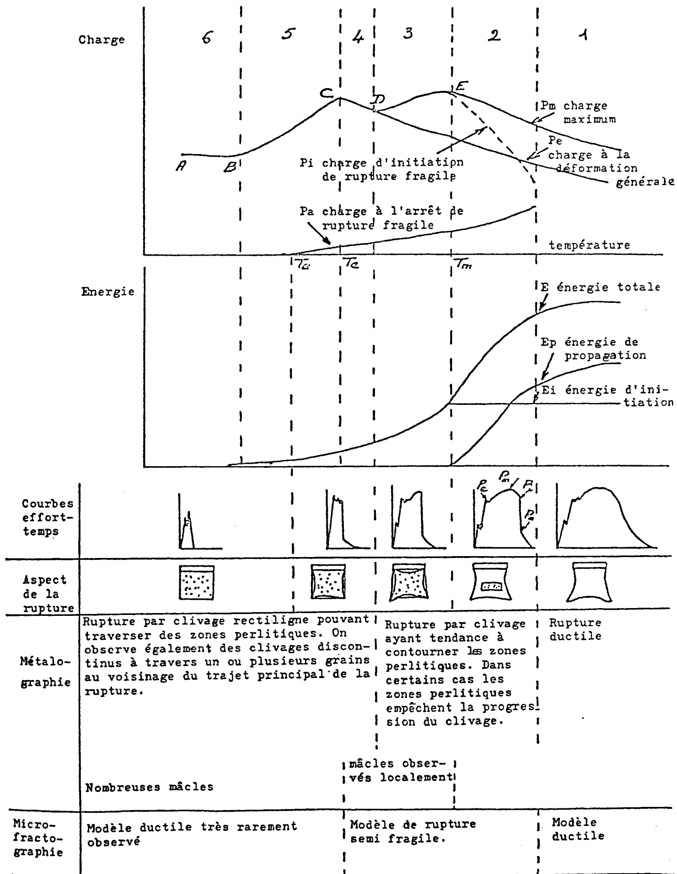
Fig. 8 : Tableau synoptique des résultats des essais CHARPY obtenus pour des températures variables dans la zone de transition
